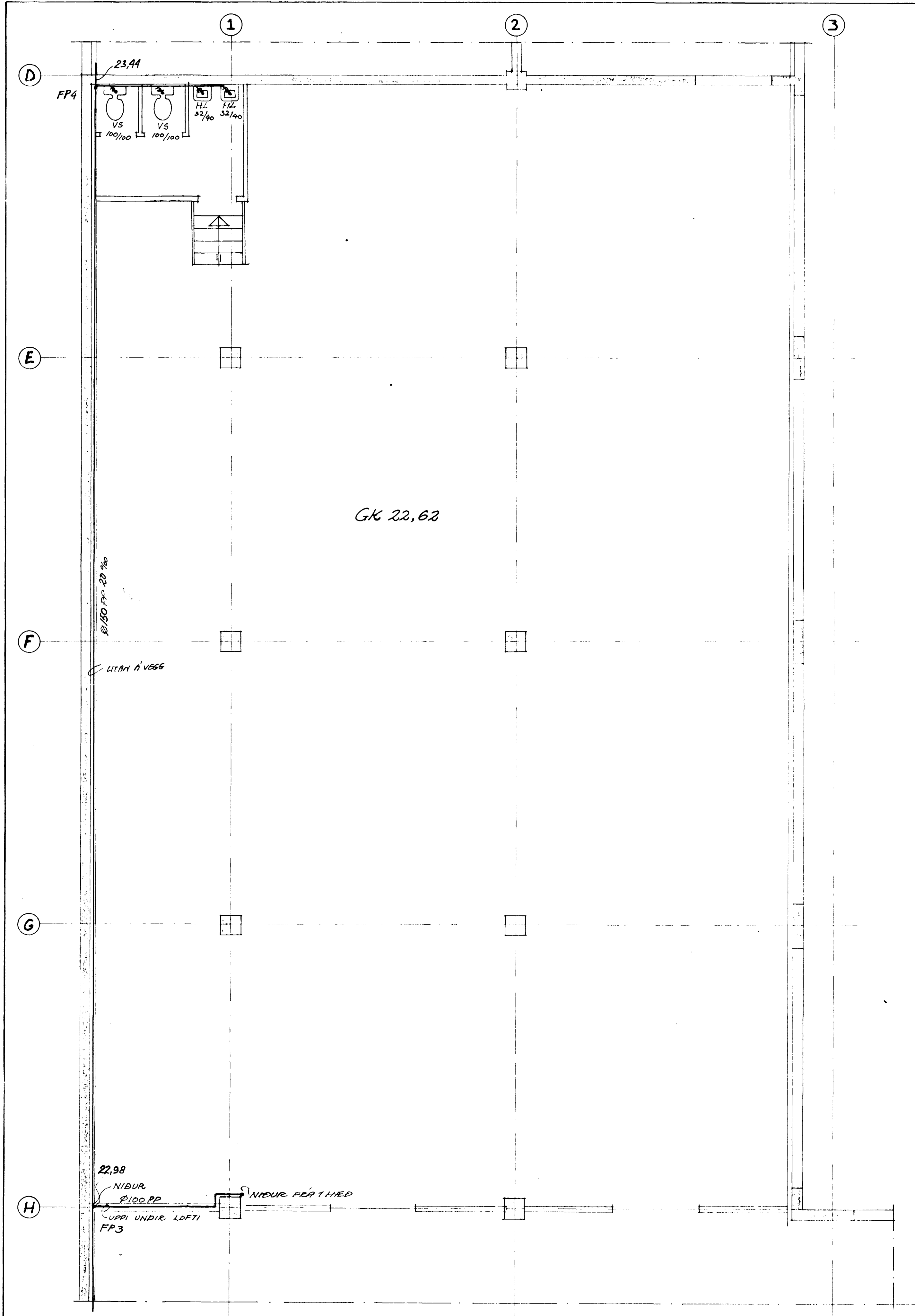
GRUNNMYND KJALLARA, HLUTI III 1:50
