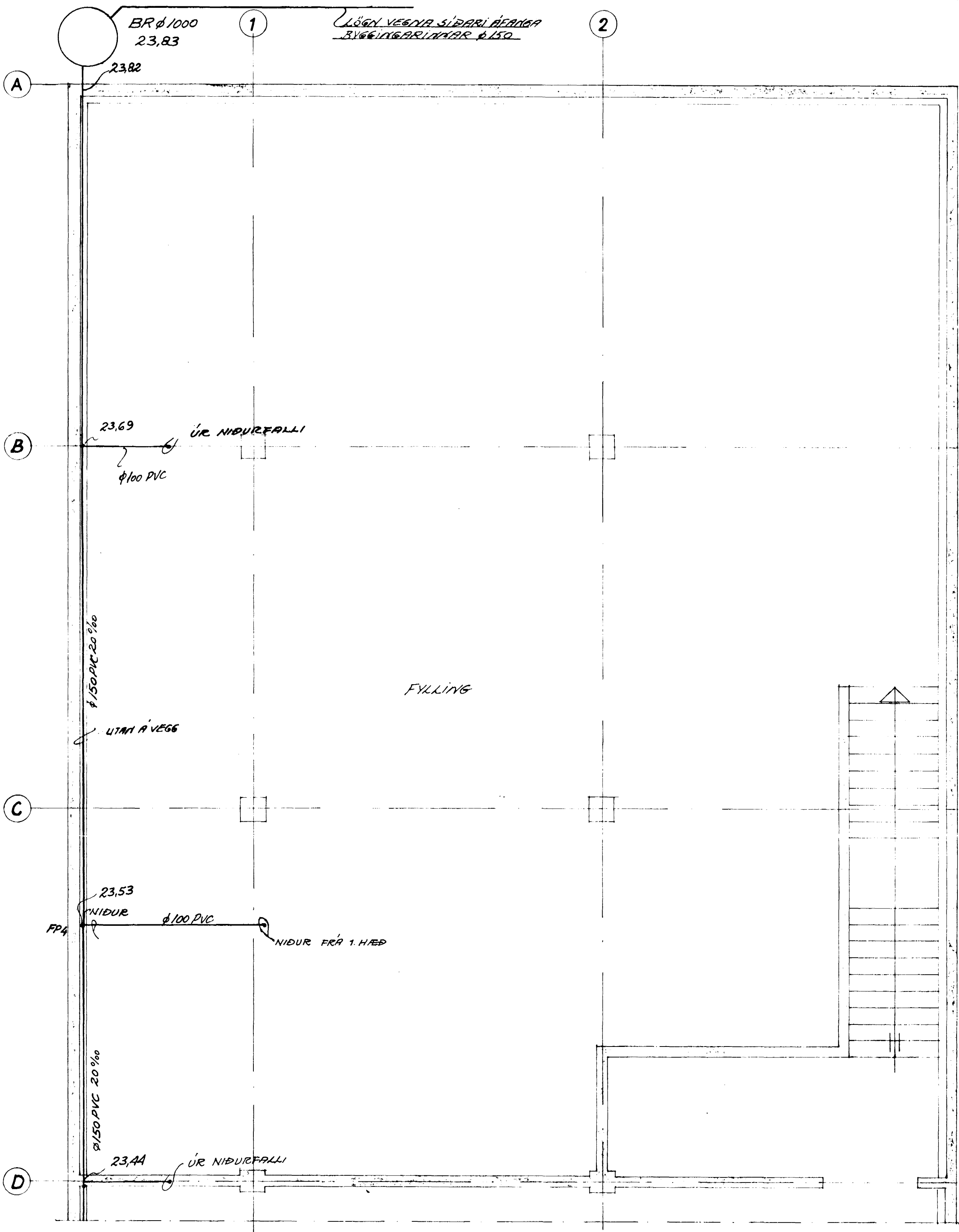
GRUNNMYND KJALLARA, HLUTI IX 1:50
