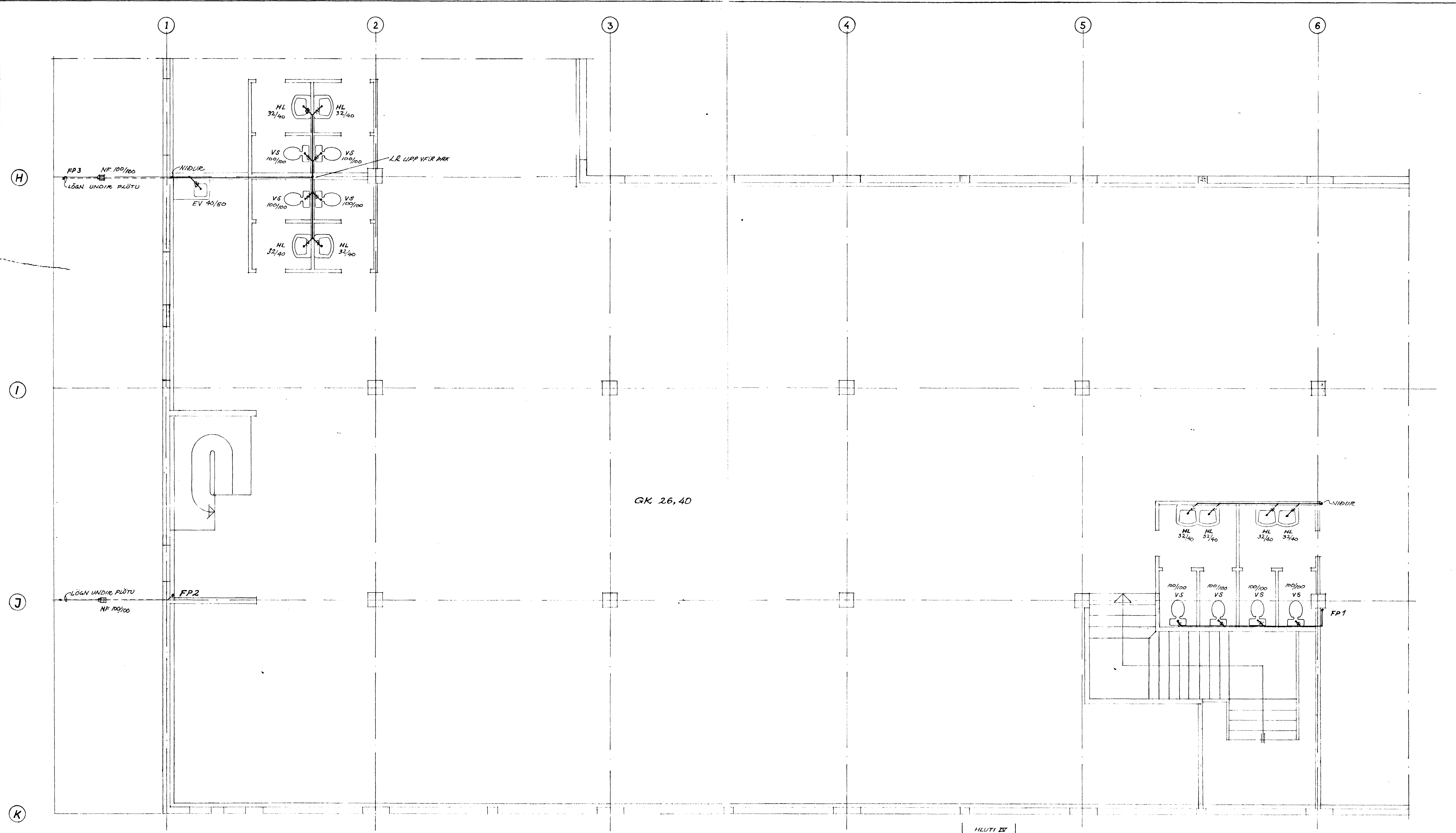
GRUNNMYND 1. HÉÐAR, HLUTI I 1:50
