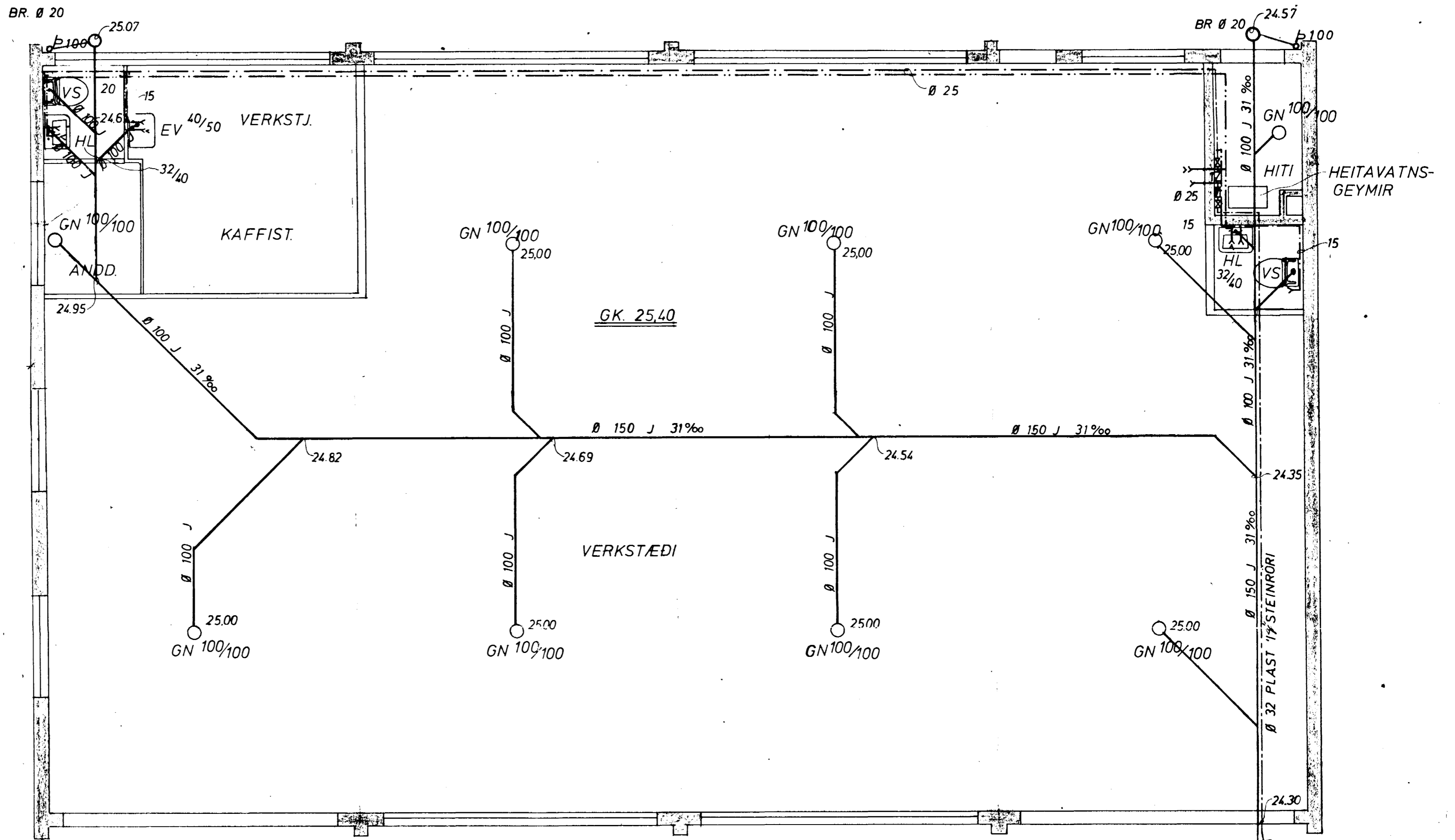
GRUNNMYND 1:50
