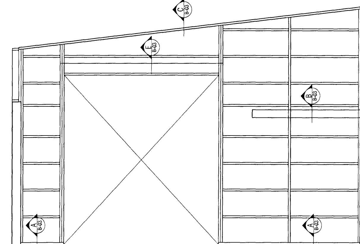
AUSTUR - veggjagindur
