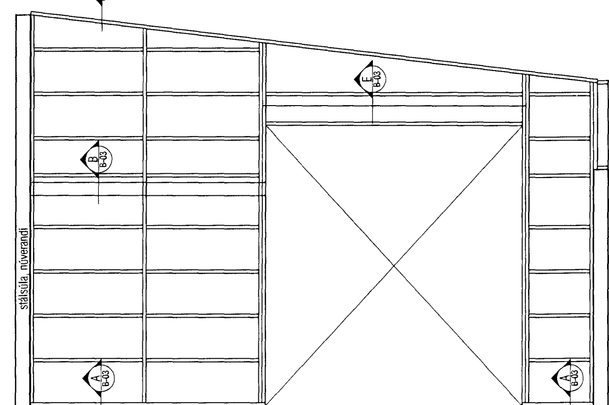
VESTUR - veggjagindur
