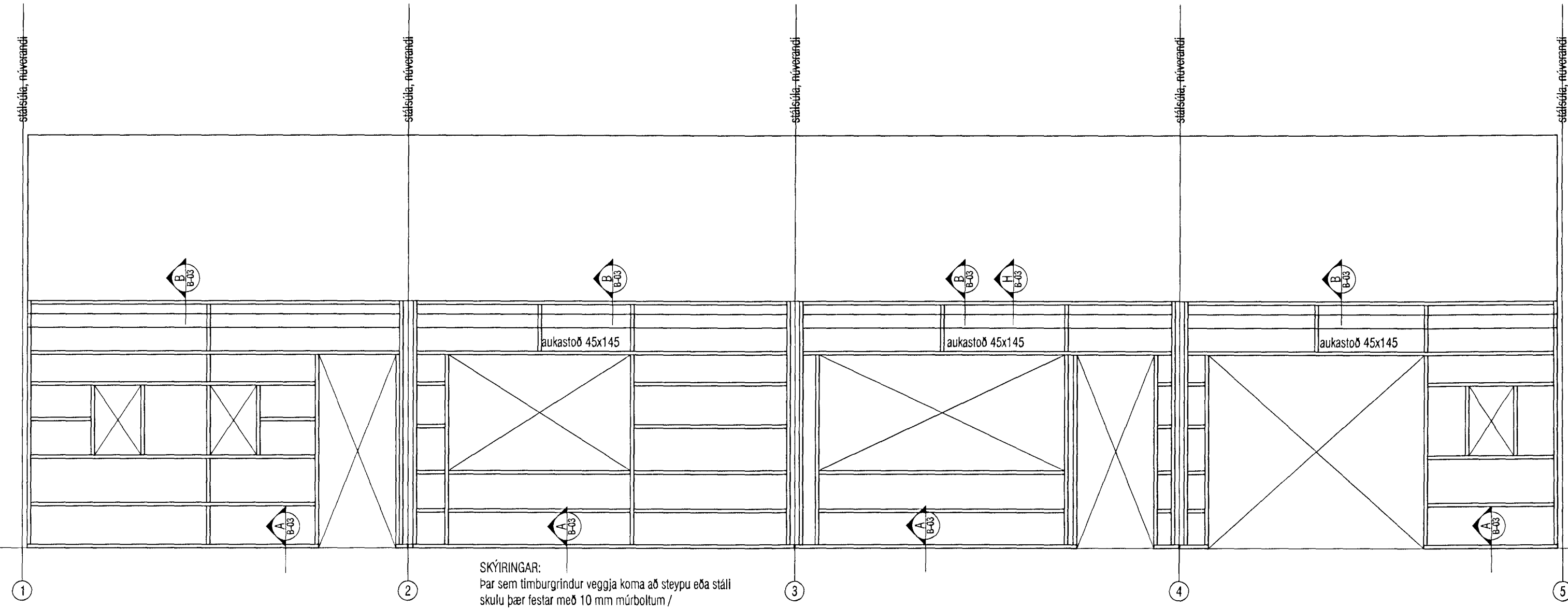
NORÐUR - veggjagindur
