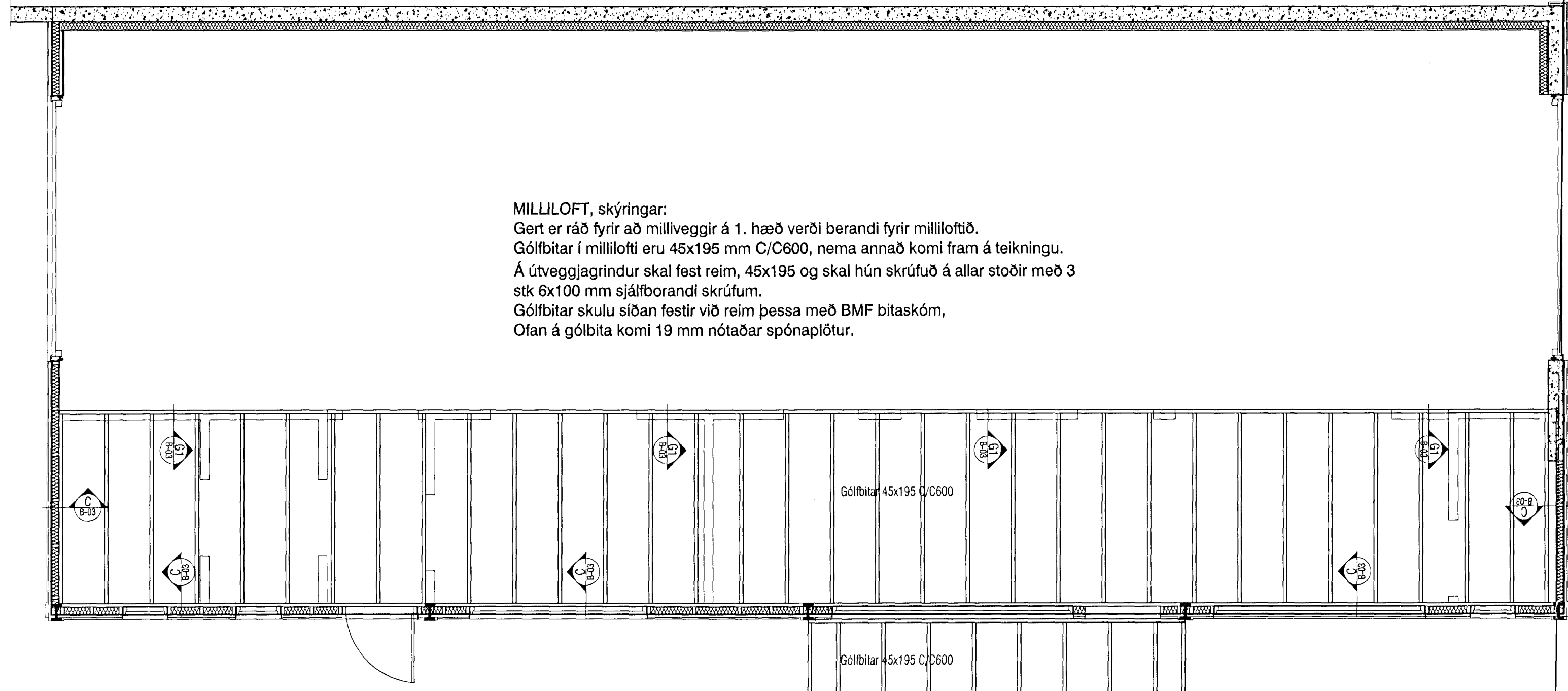
MILLILOFT - SKYGGNI
