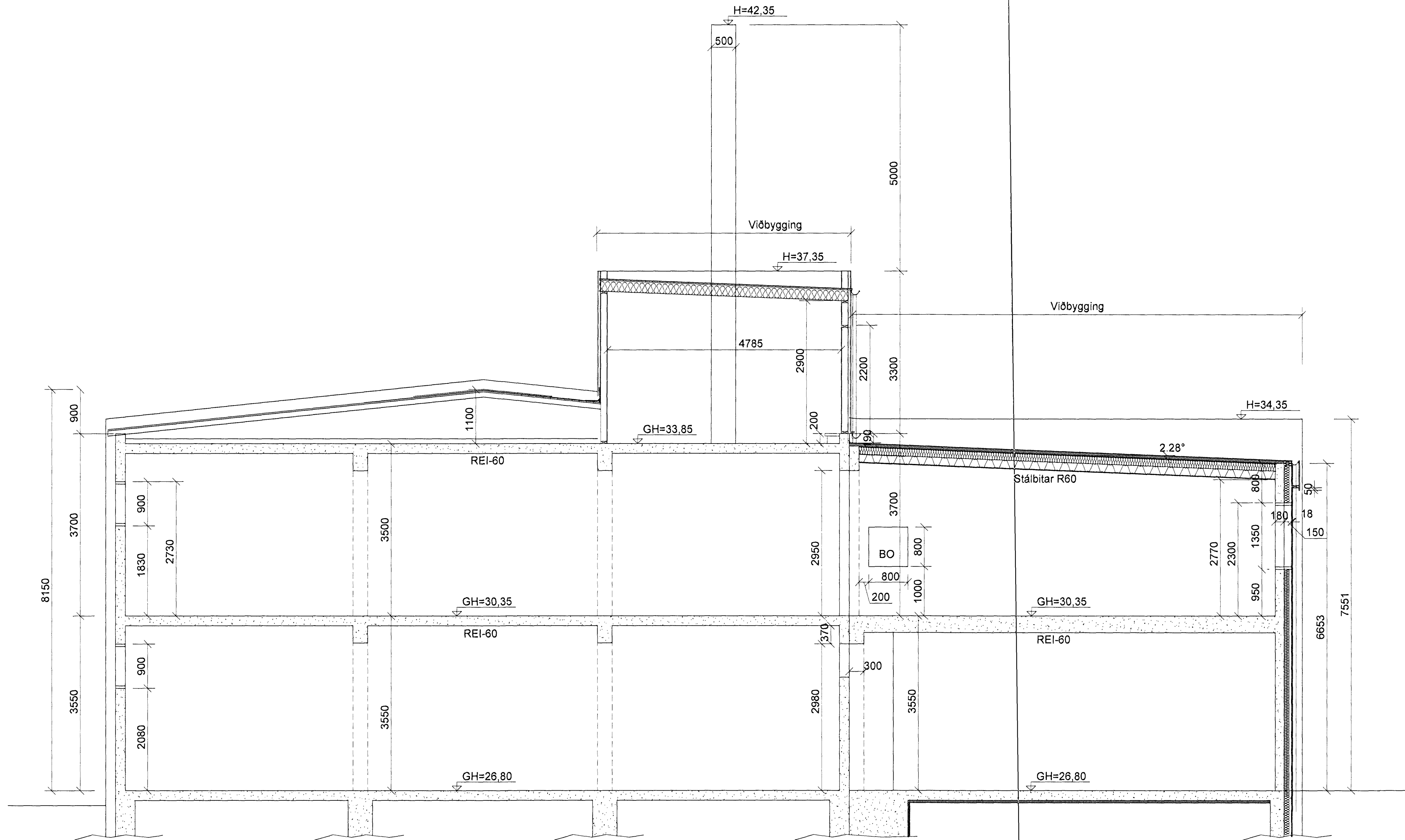
Snið A - A 1 = 100 mm
