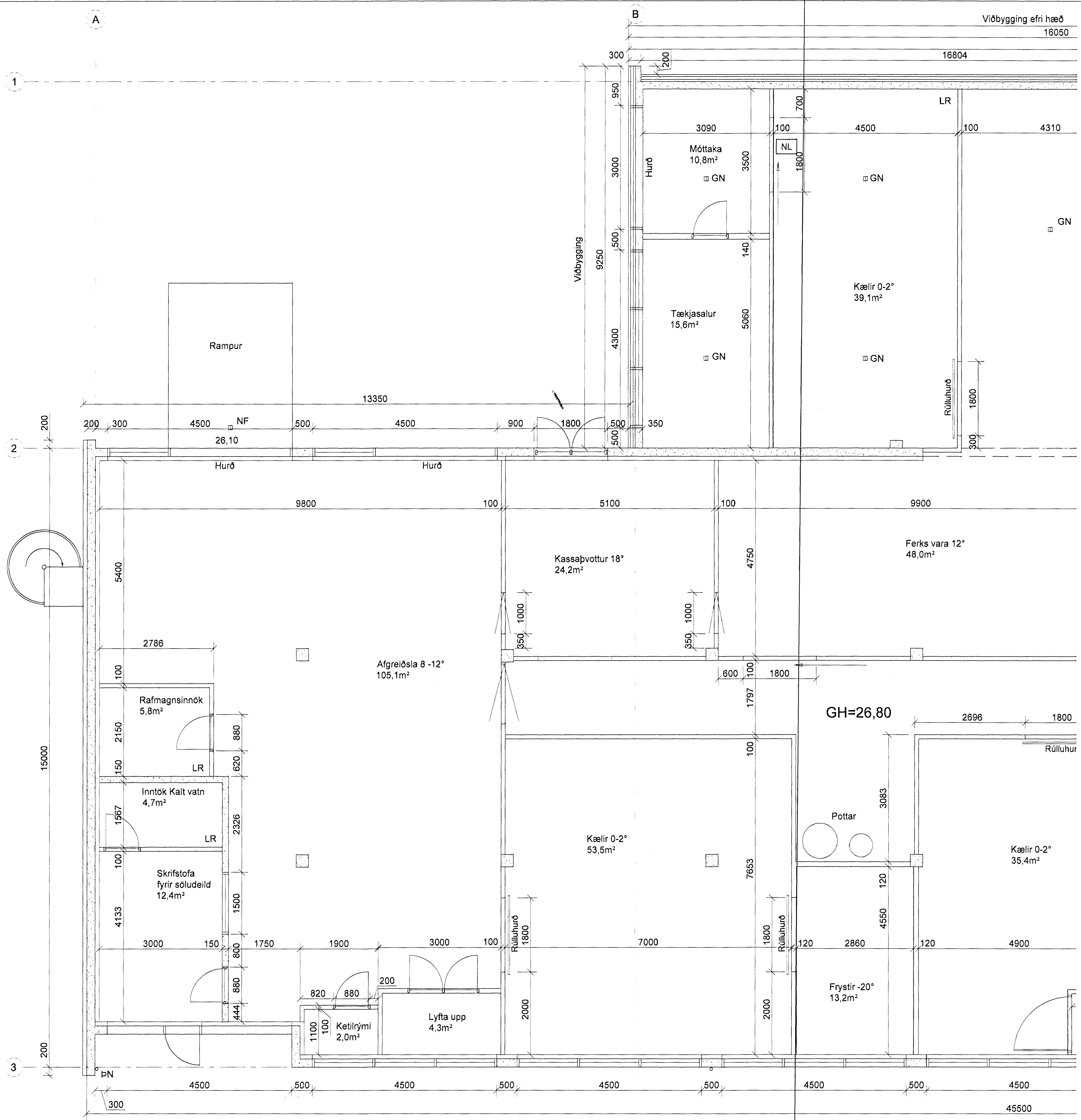
Grunnmynd 1, hæð 1 = 100 mm
