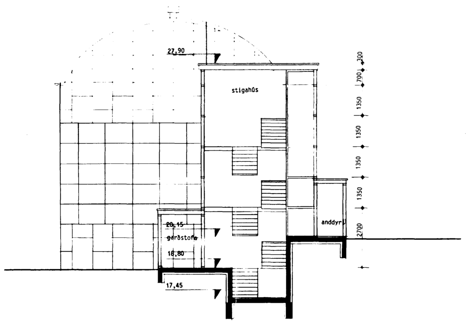
SKURÐUR B - B
