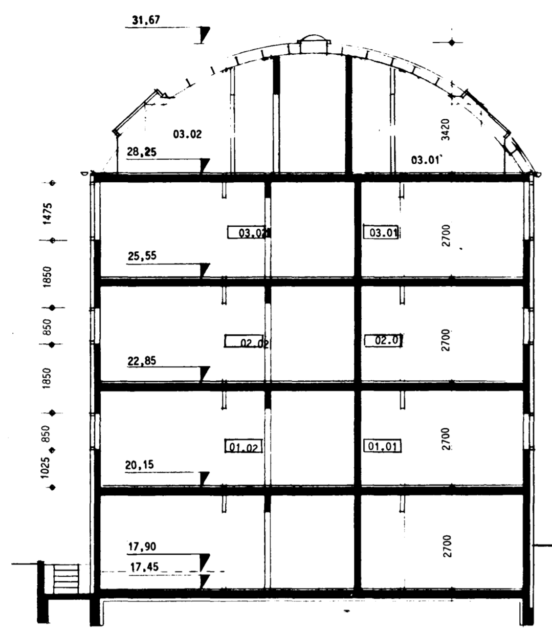
SKURÐUR C - C
