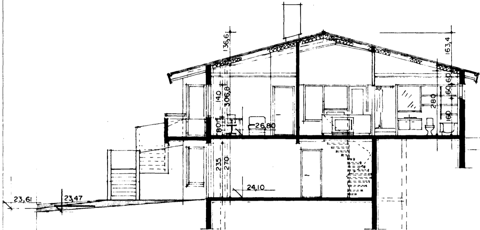
SNEIÐING A - A MKV. 1:100
