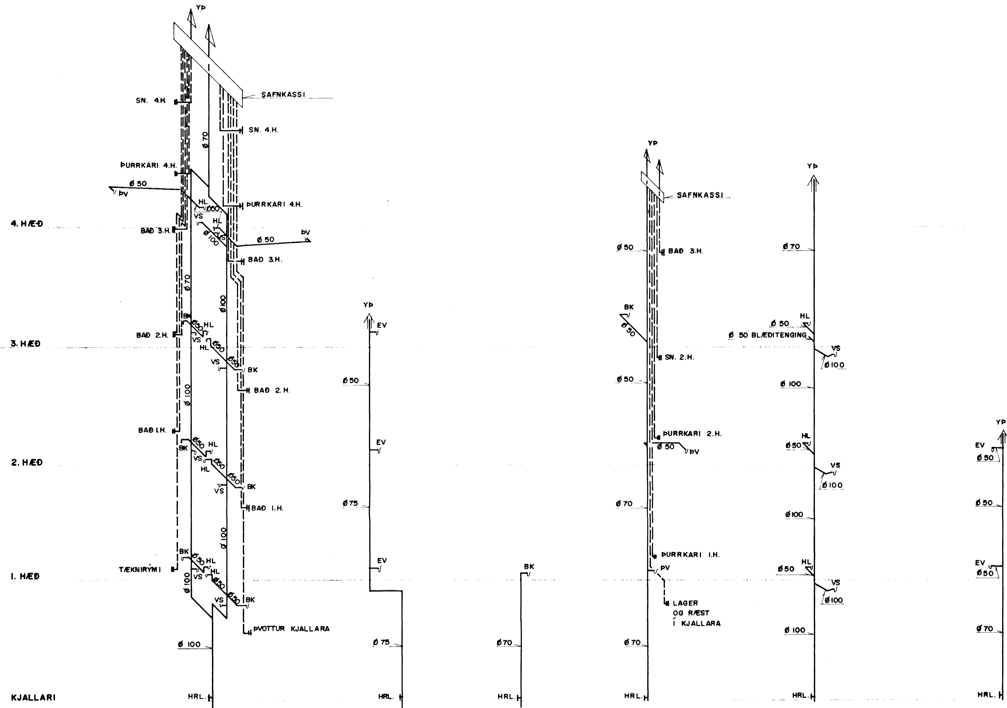
FALLPÍPA Fp. 1 Fp. 1a / Fp. 1b
