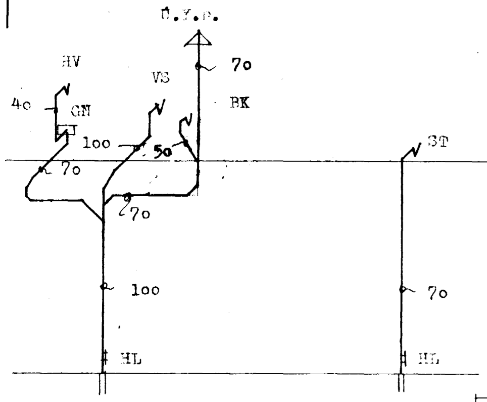
STOFN A 1:50
