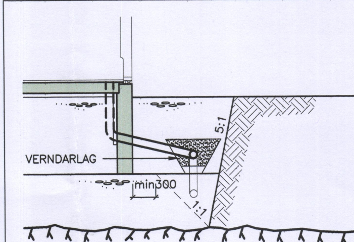
SNID VÍÐ SÖKKUL Mkv. 1:50
