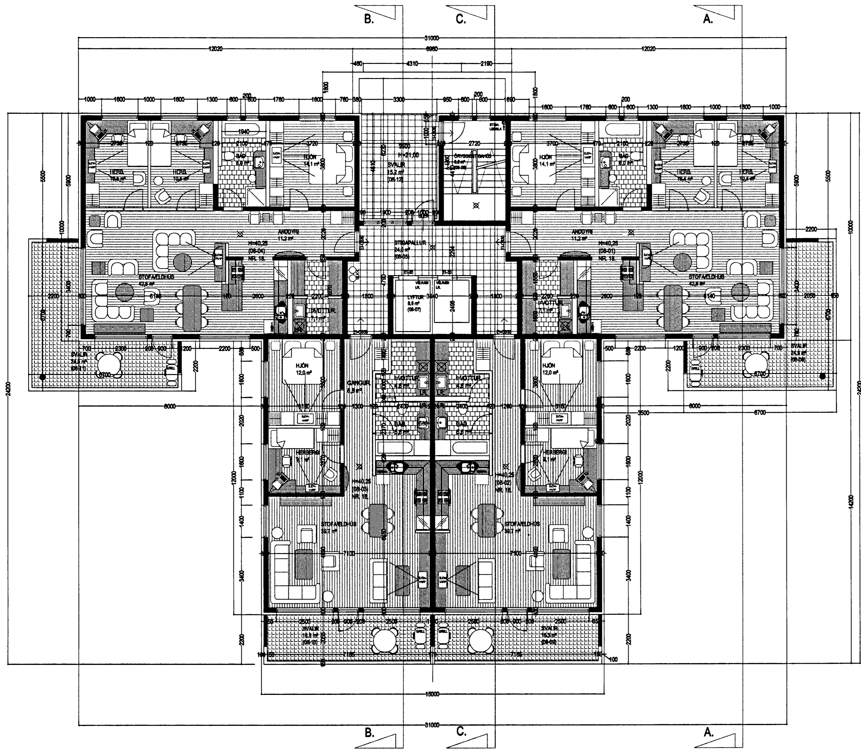
GRUNNMYND 8. HÆÐ MKV. 1:100.
