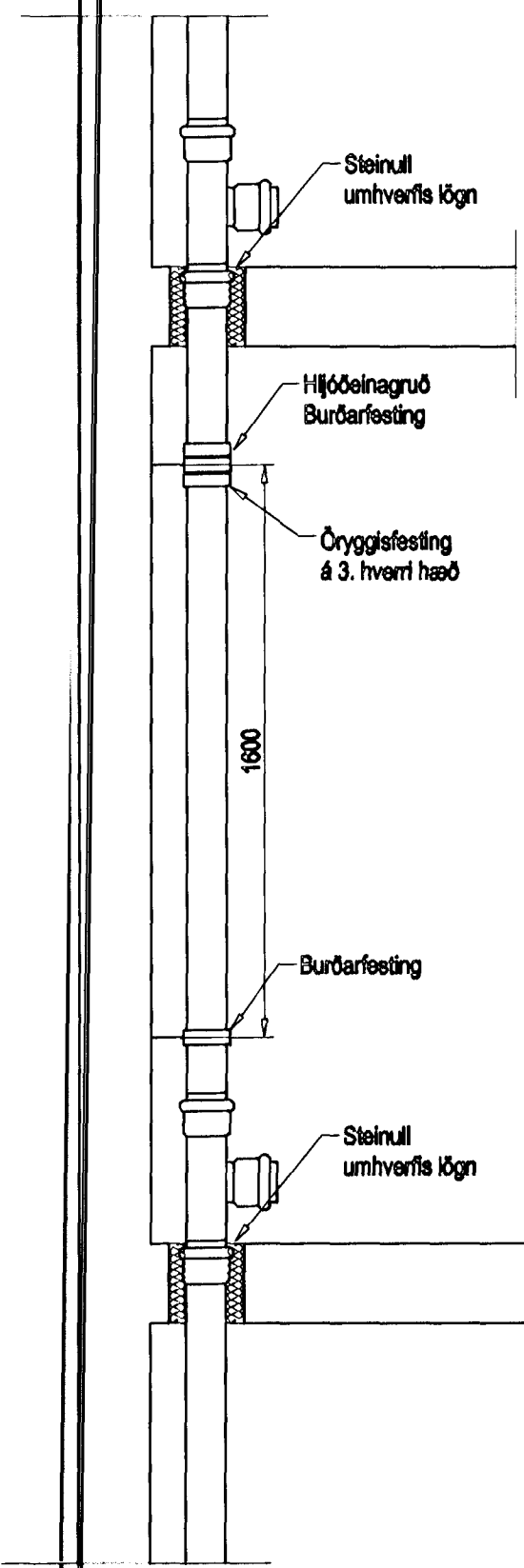
Fallþípa, festingar 1:20
