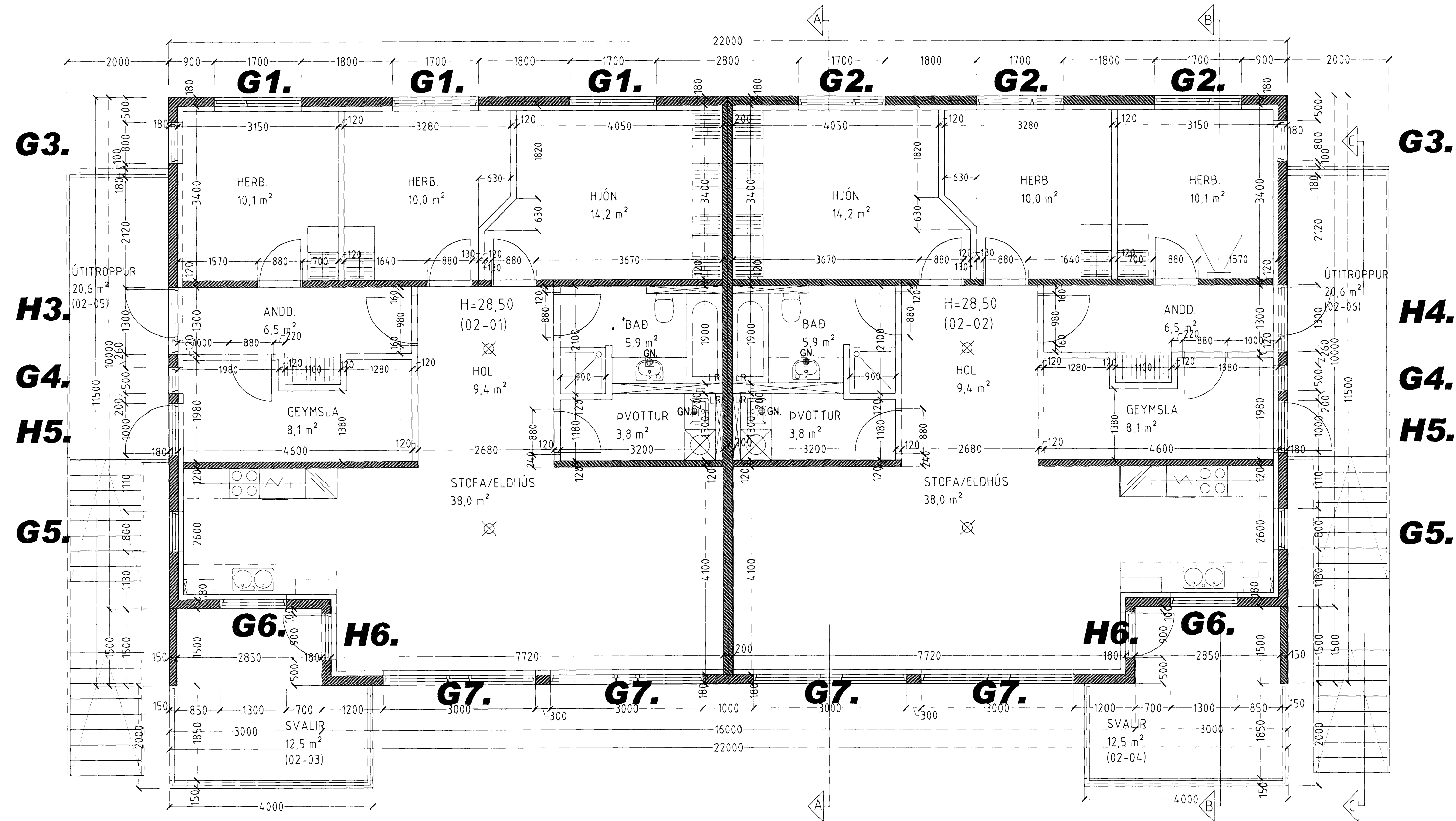
GRUNNMYND 2. HÆÐ MKV. 1:50.
