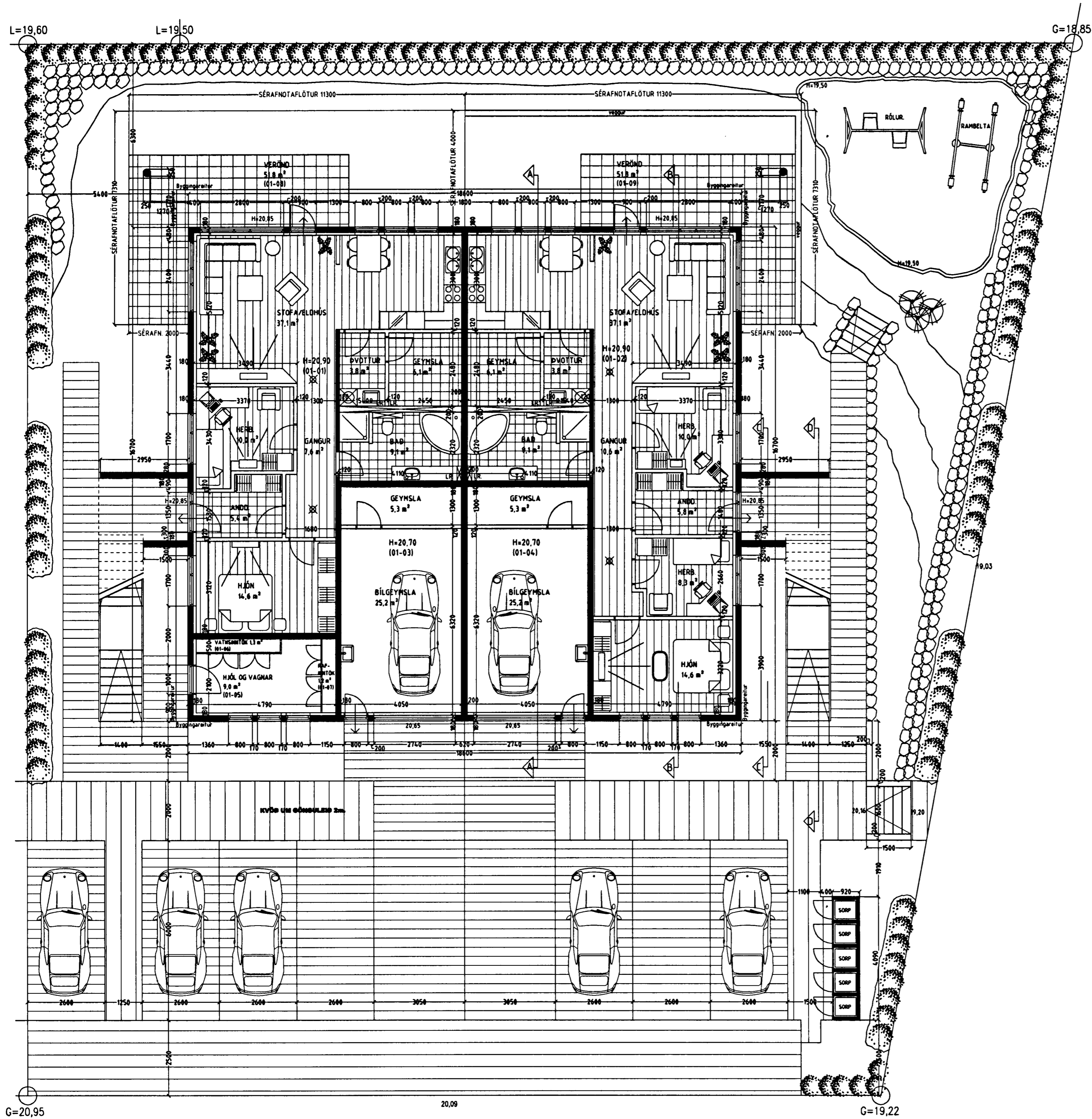
GRUNNMYND 1. HÆÐ MKV. 1:100.
