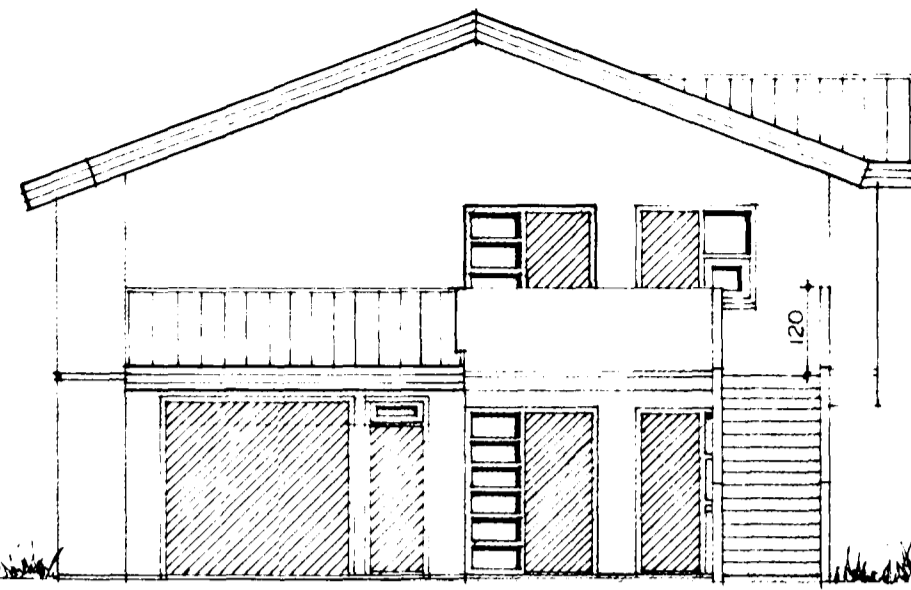
ÚTLIT NORDUR MKV. 1:100.
