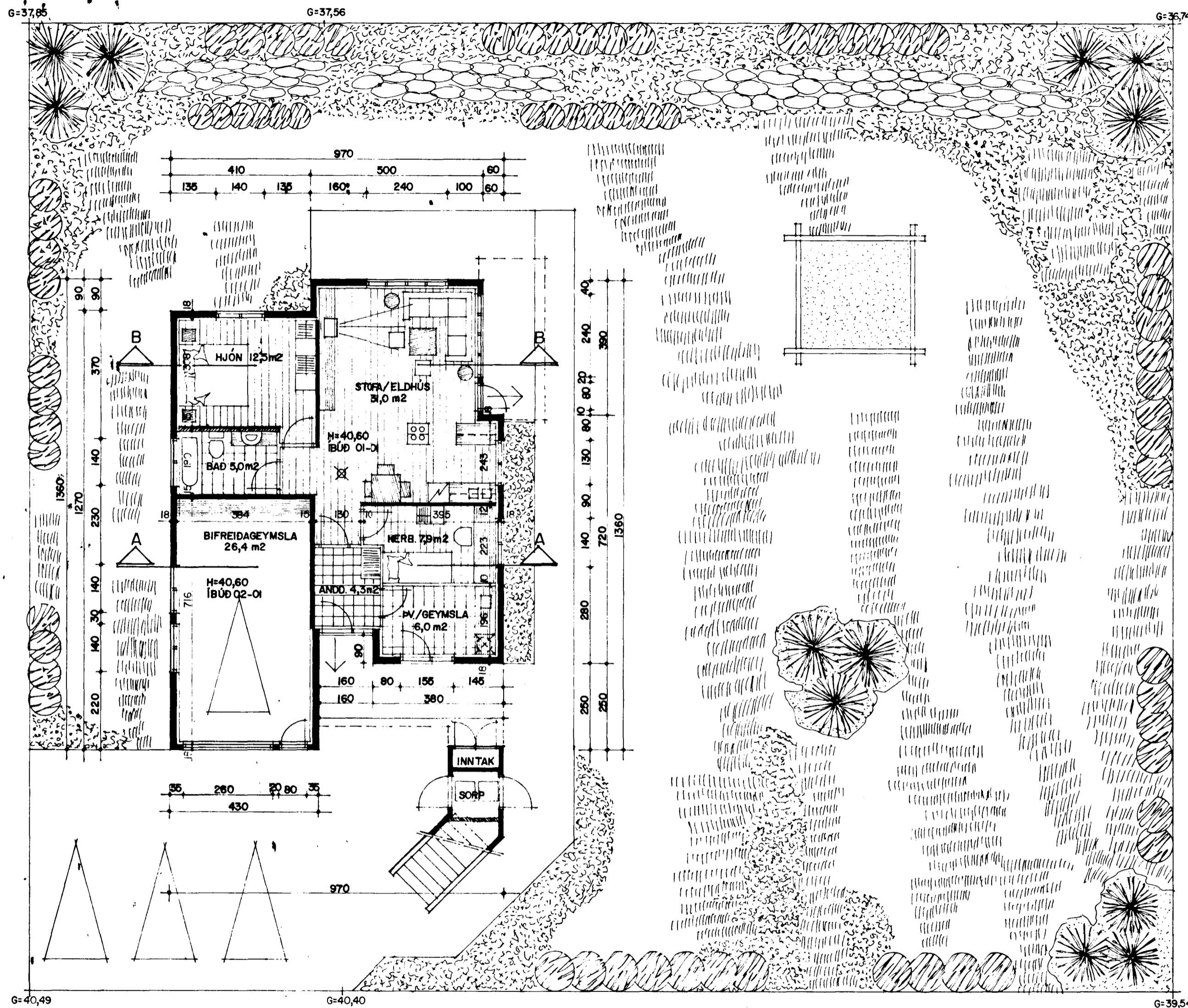
GRUNNMYND I HÆÐ MKV. 1:100.
