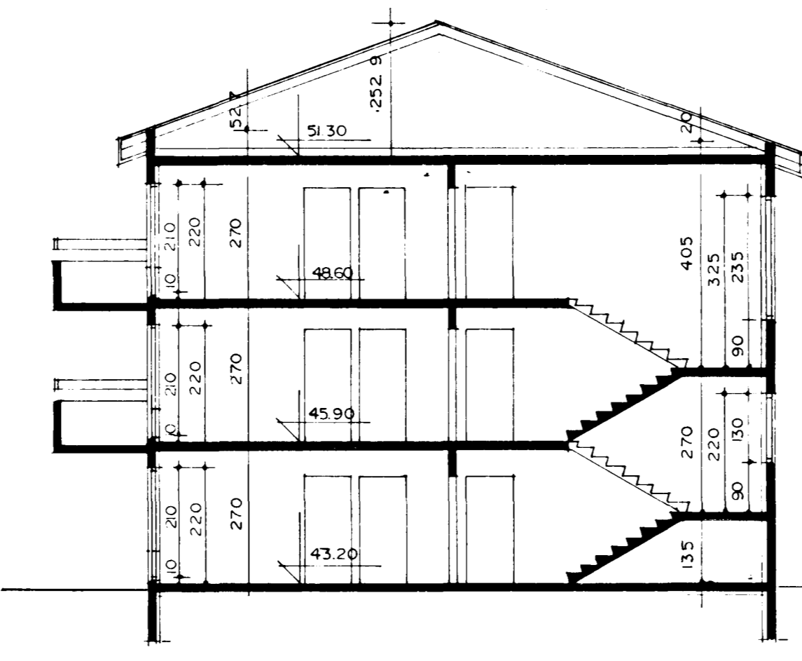
SNID A-A MKV 1:100
