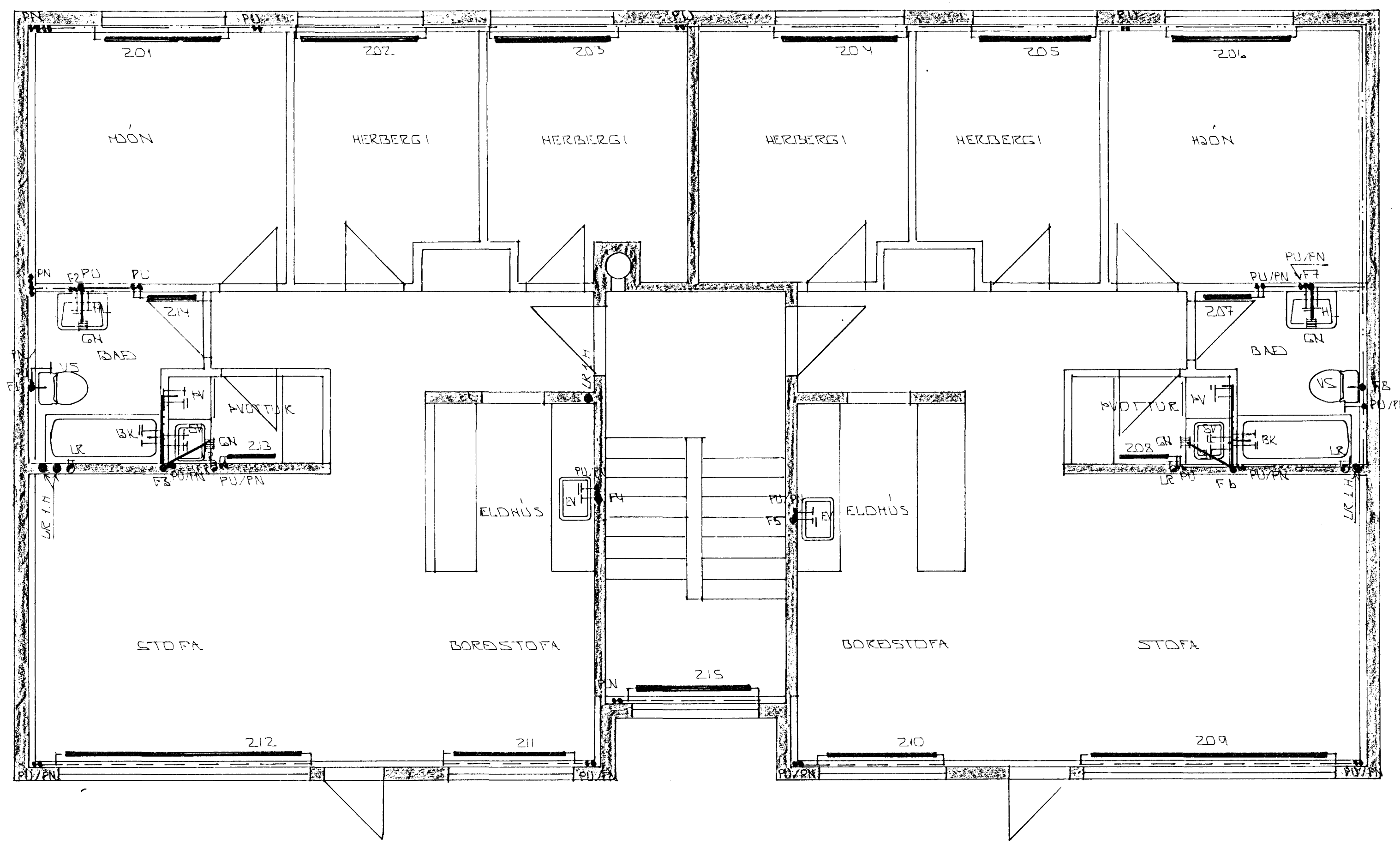
GRUNNMÝND 2. HÆÐ 1:50
