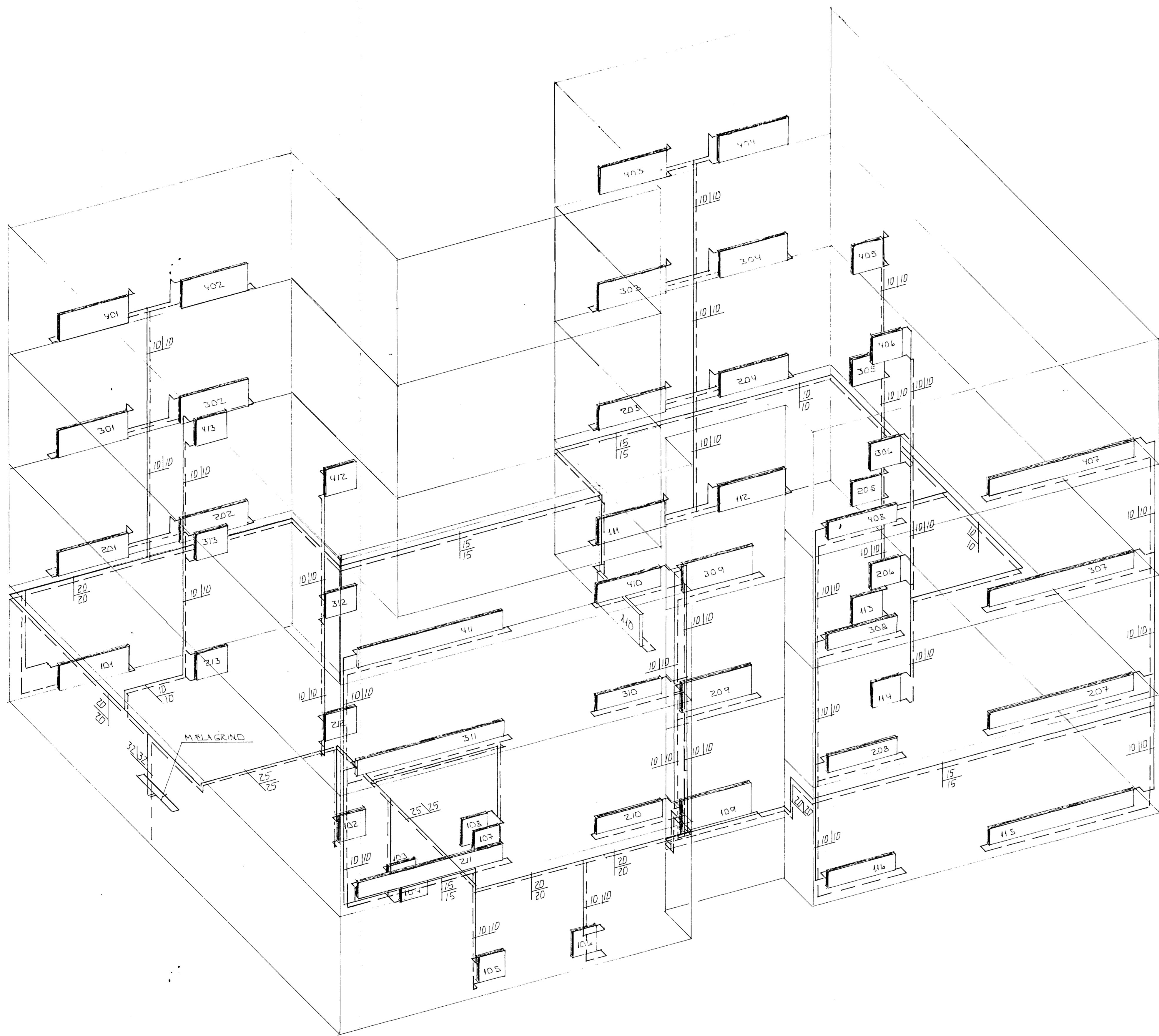
RÚMMYND HITALAGNA ~1:50
