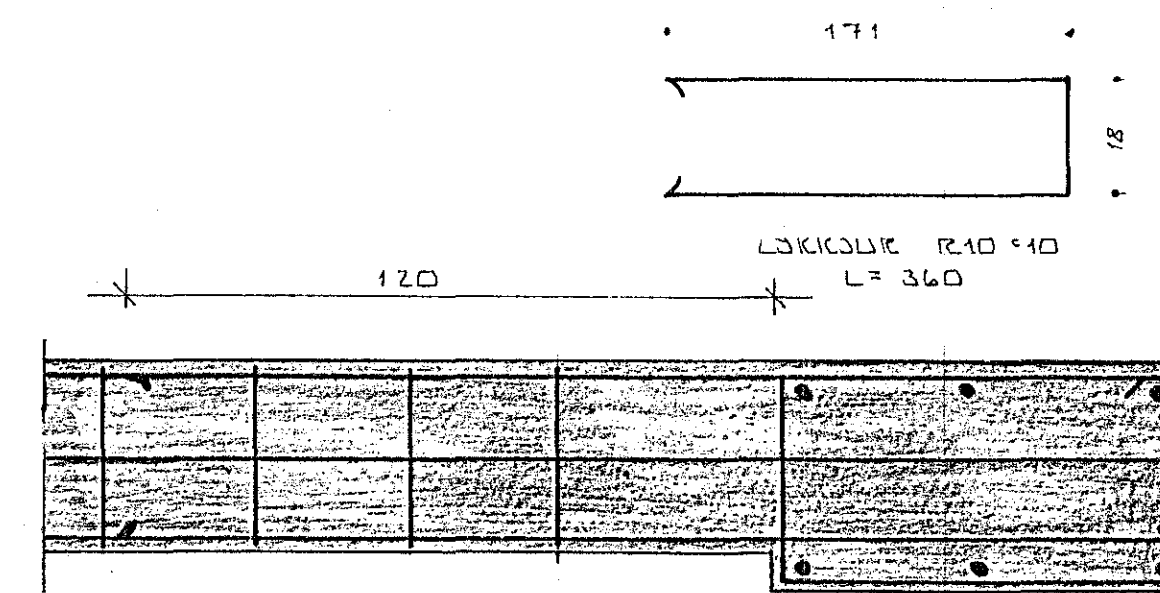
SNID D-D 1:10
