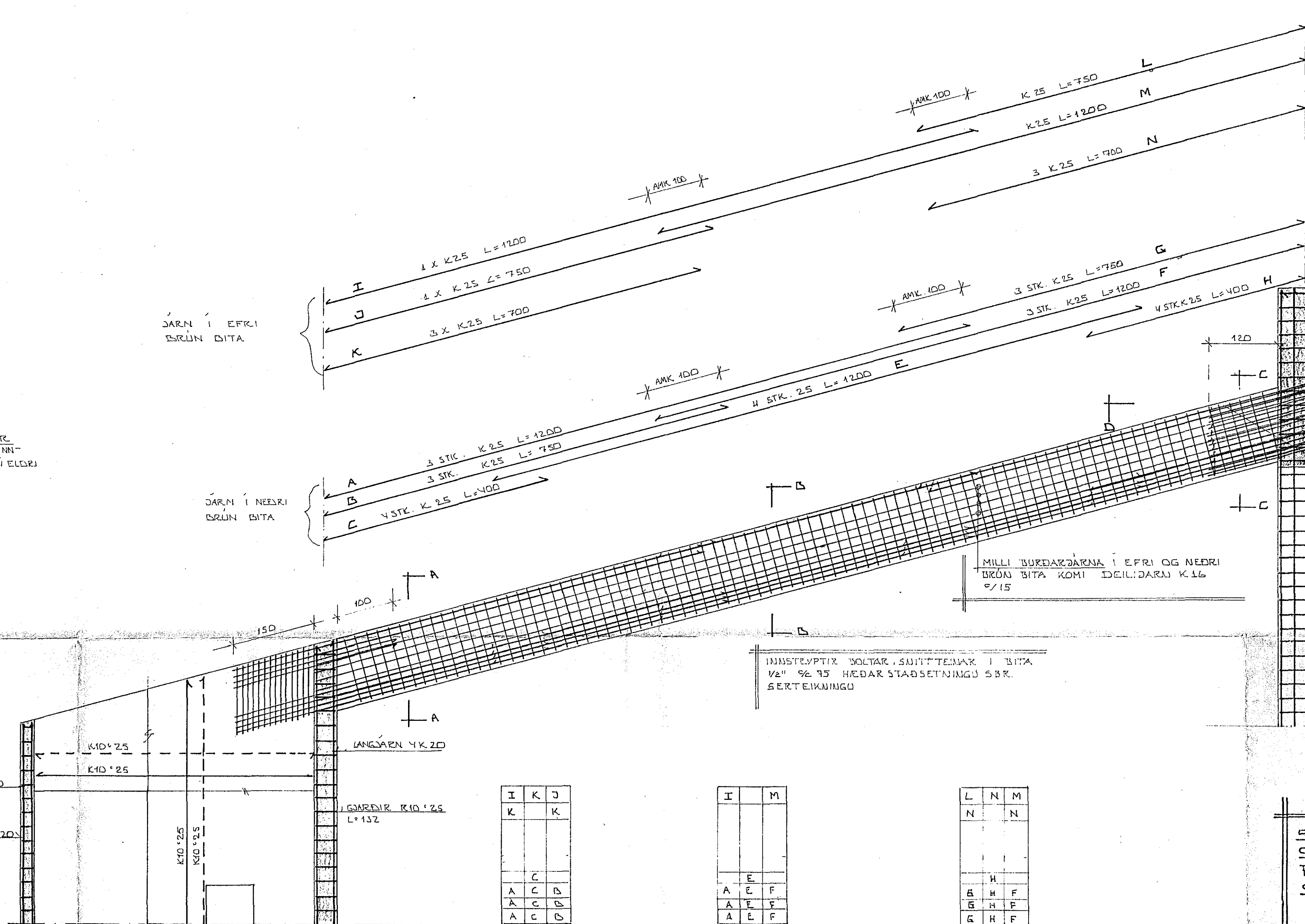
SNID A-A STAÐSETNING JÄRNA Í BITA
