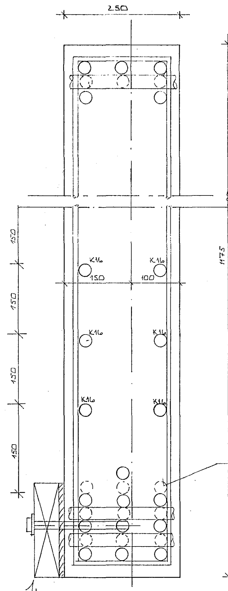
SNID I BITA 1:5 STAÐSETNING JÄRNA Í BITA.
