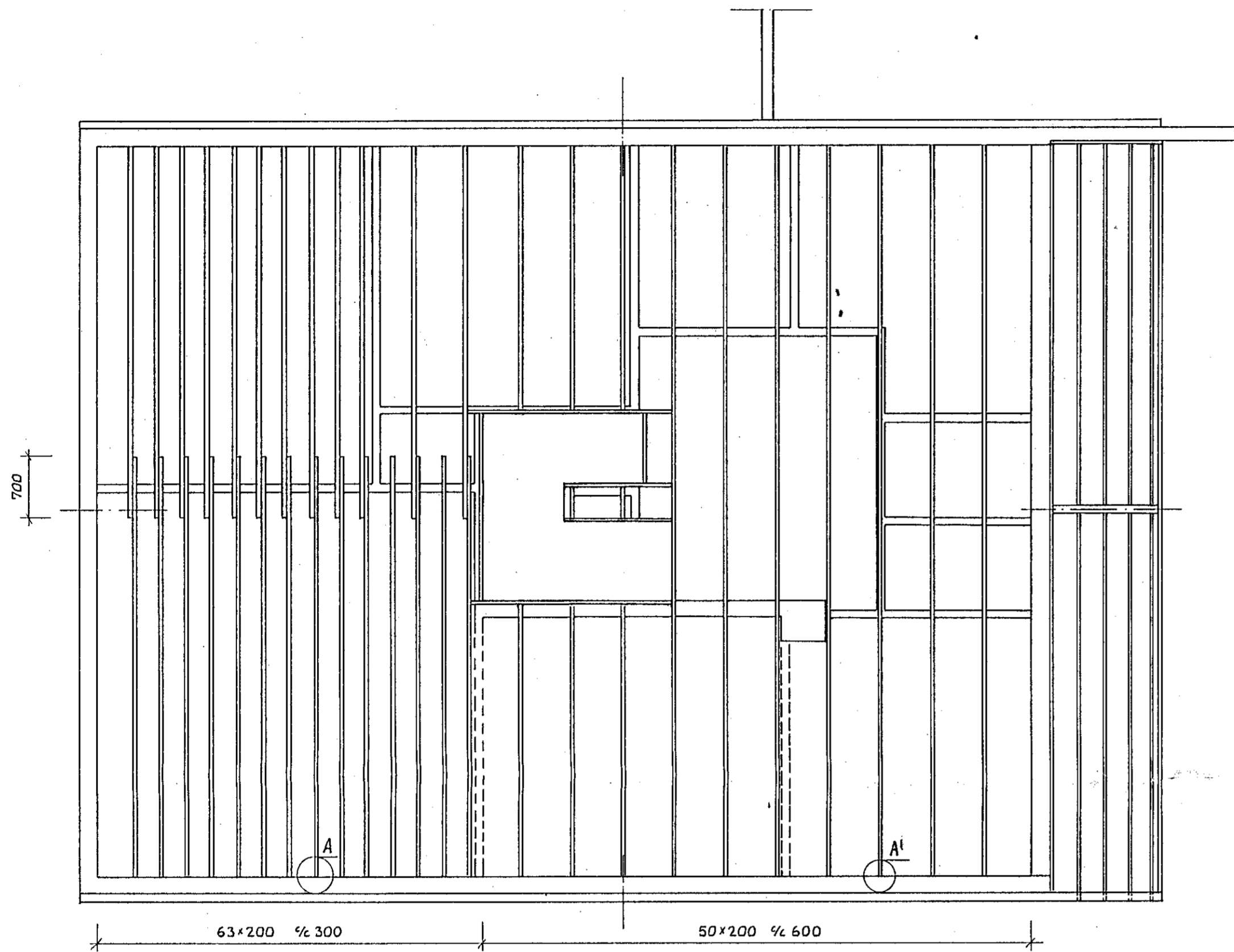
STYRKING GÓLFS RISHÆÐAR 1:50
