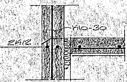
SKURÐUR E, M=1:20
