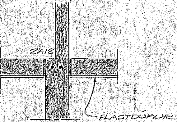
SKURÐUR C, M=1:20
