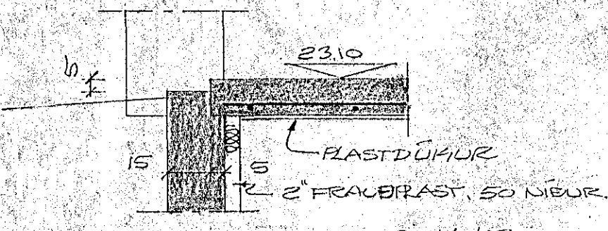
SKURÐUR B, M=1:20
