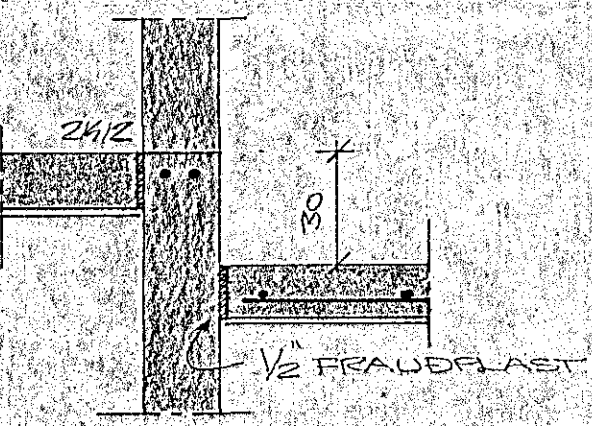
SKURÐUR D, M=1:20
