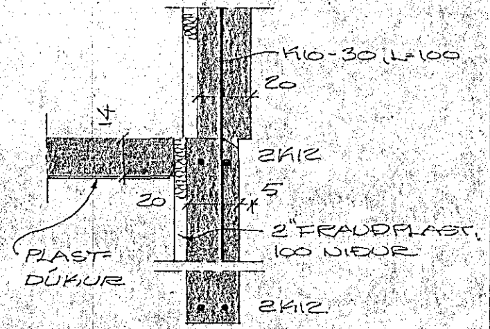
SKURÐUR A1, M=1:20
