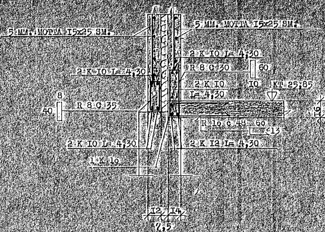
SNID D-D 1:20
