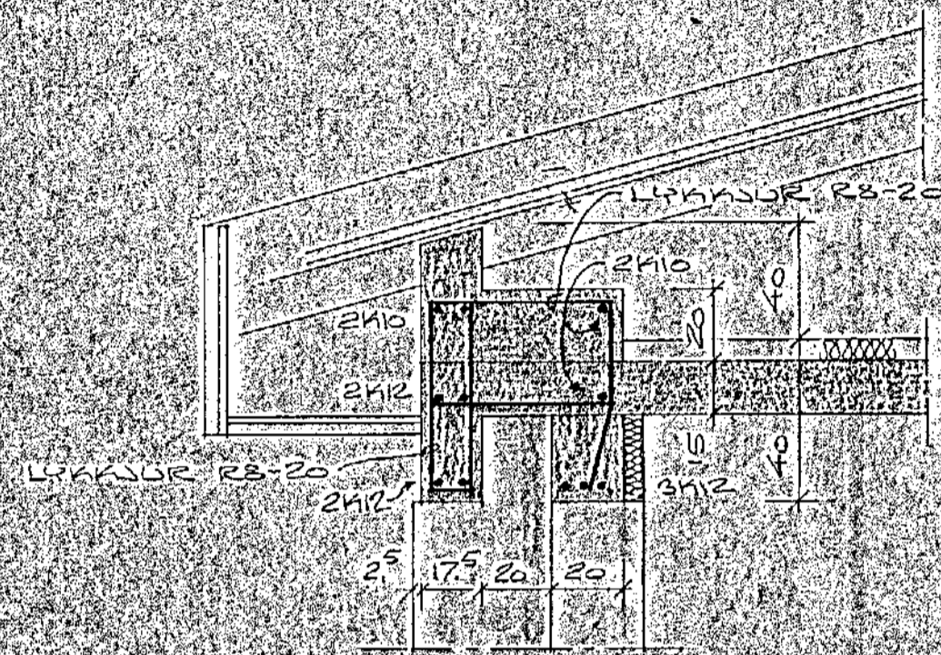
SKURÐUR E. M. 1:20
