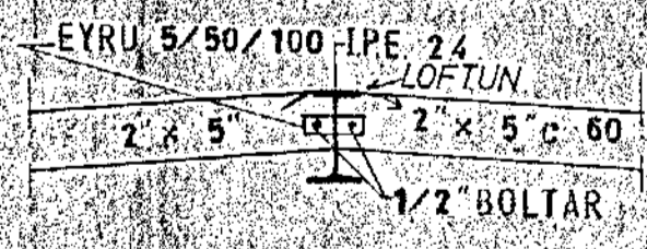
SNID D 1:20
