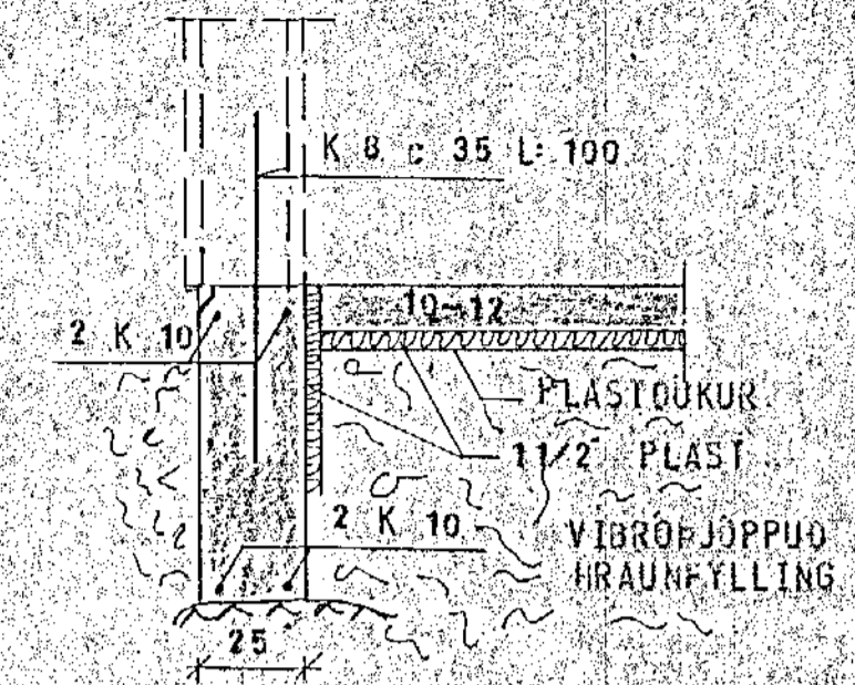
SNID 'I ÚTVEGG 1:20
