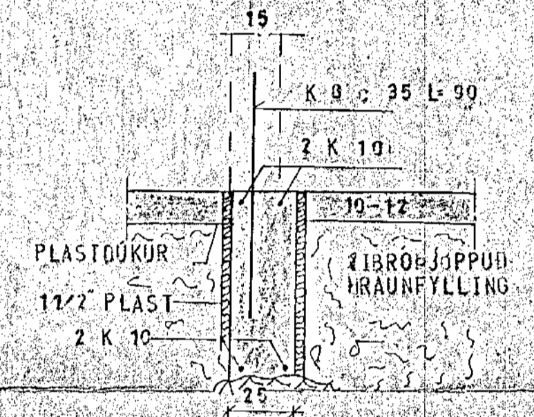
SNID 'I INNVEGG 1:20
