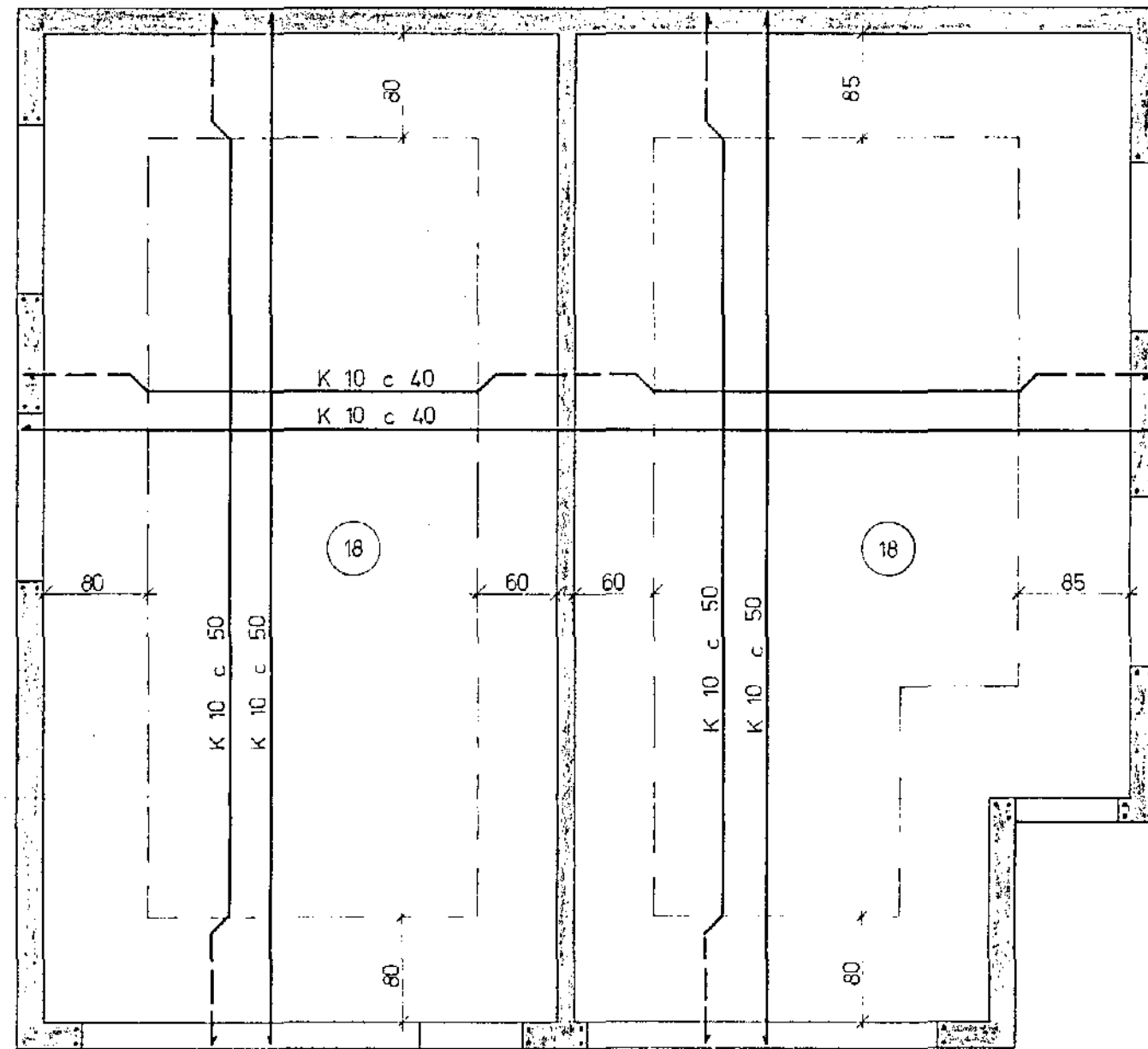
GRUNNMYND 1 : 50
