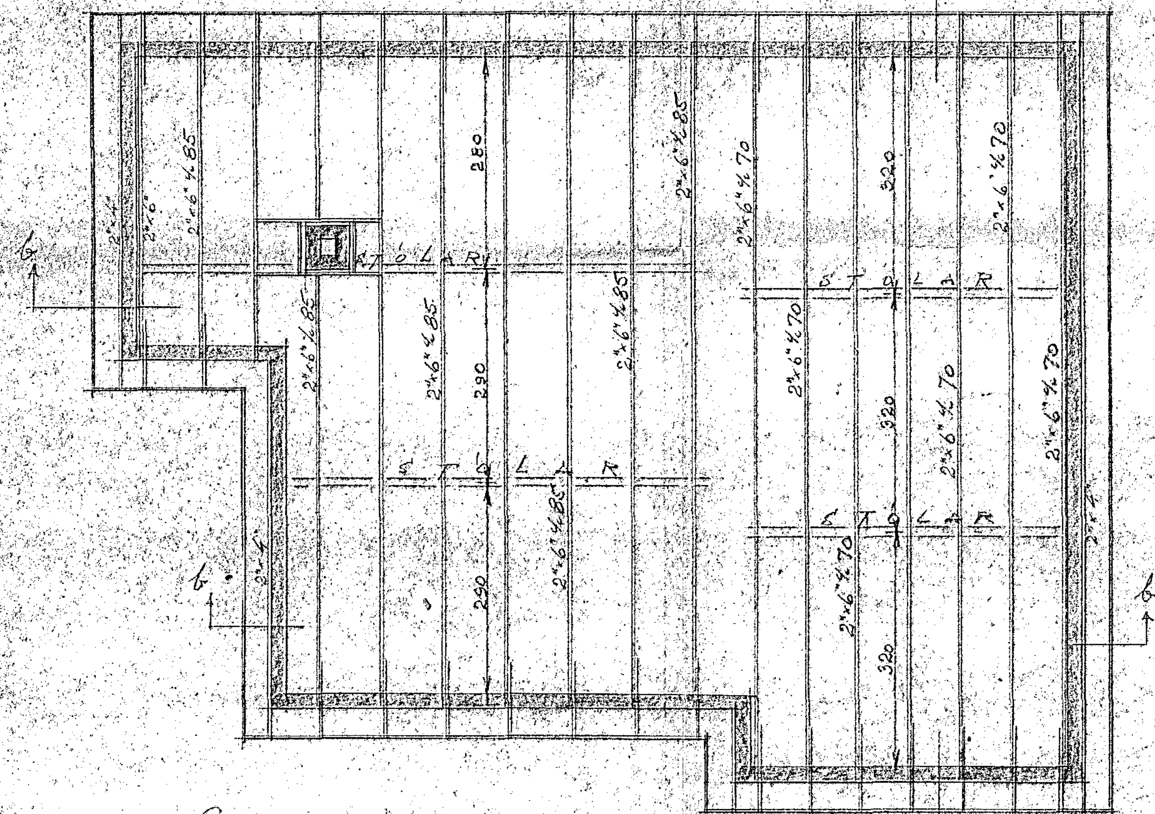
GRUNNMYND KVARNI 1:50
