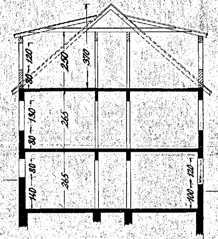
Þverskurður
