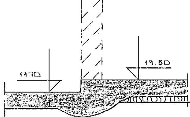
SNID 3 ~ 1:20
