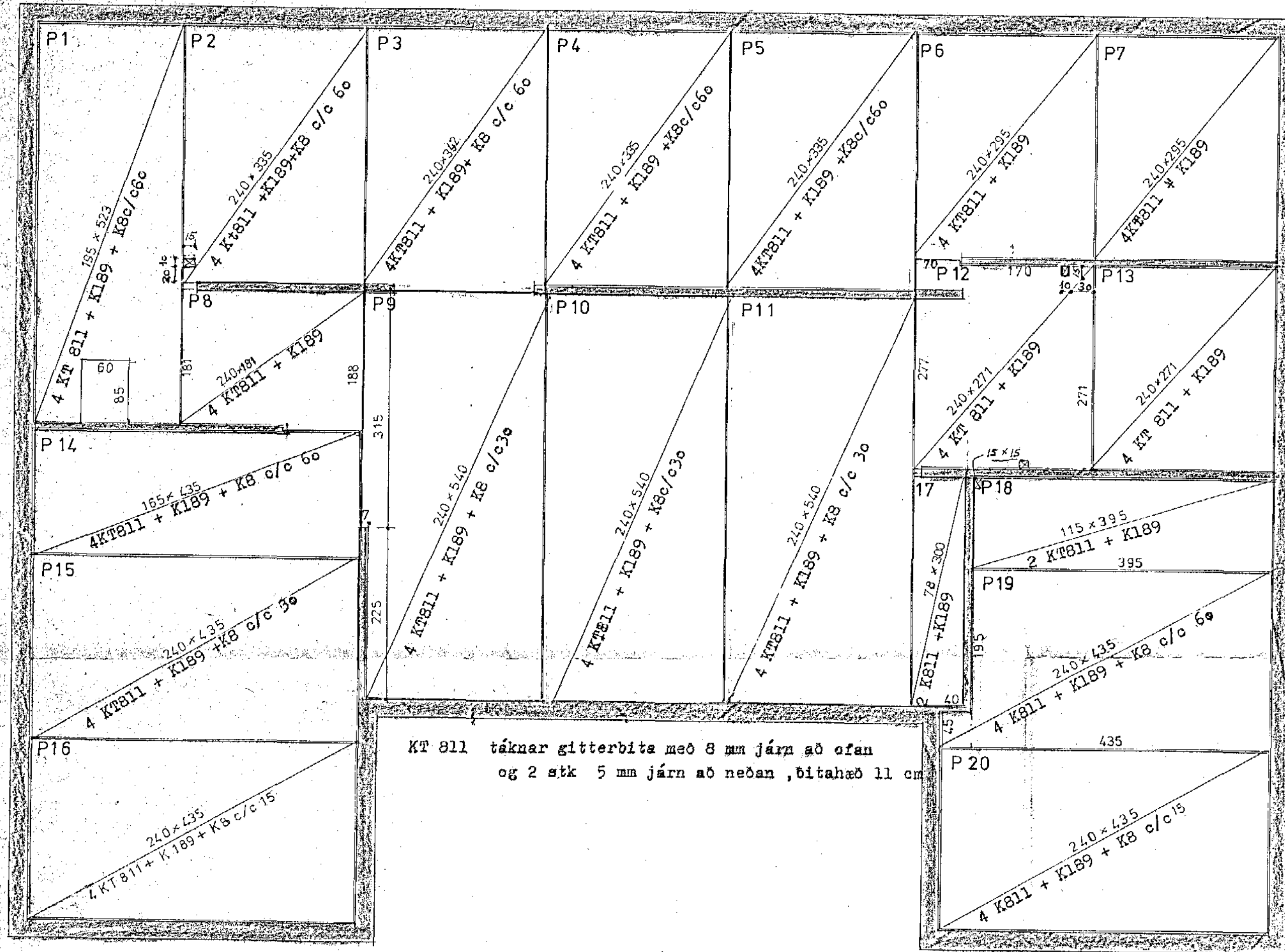
Bingaplötur í loftaplötu grunnmynd, M= 1:50
