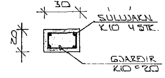
SÚLA 2 1:20
