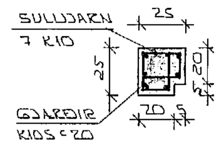
SÚLA 1 1:20
