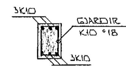
X 1:20
