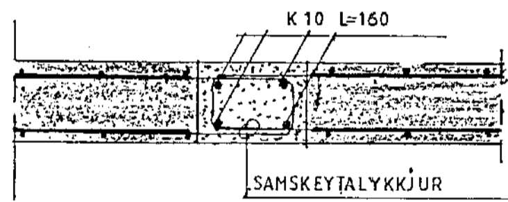
SNÍÐ A-A M;1:10
