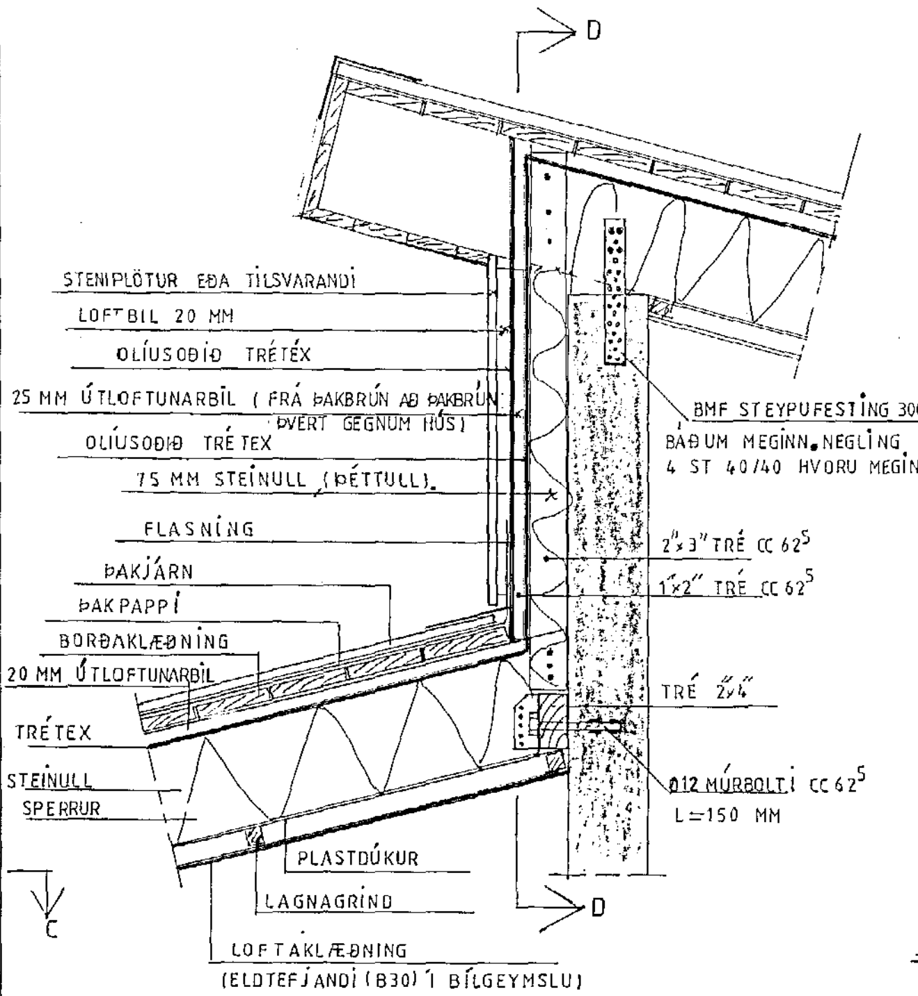
SNÍÐ B-B M: 1:10
