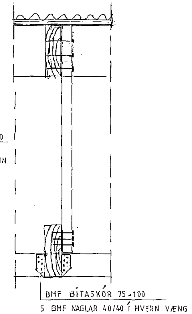
SNÍÐ D-D M: 1:10
