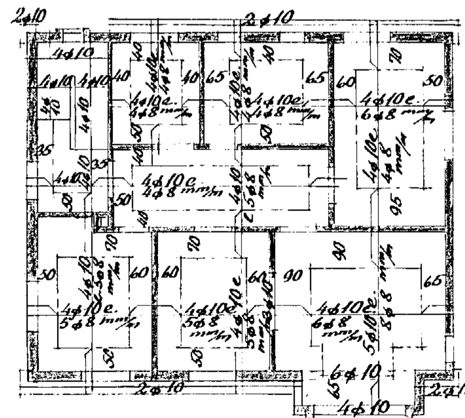
Loft yfir 2. hæð 1:100
