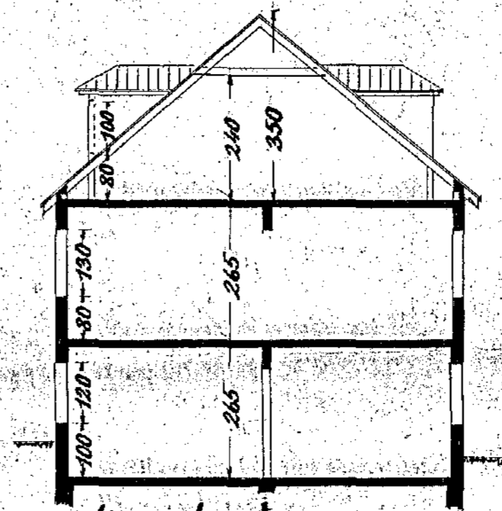
Þverskurður
