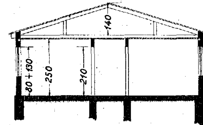
Sneiðing
