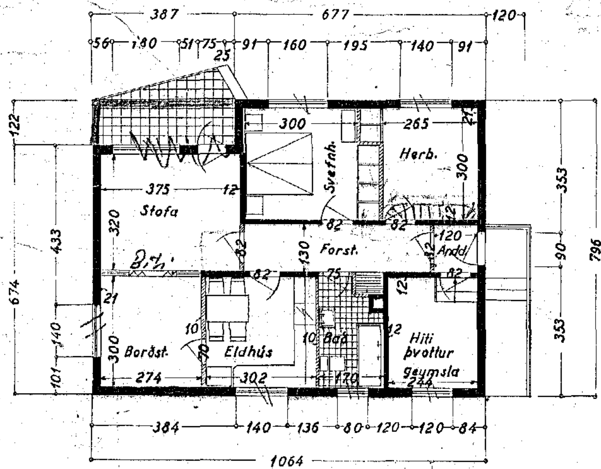
Grunnmynd
