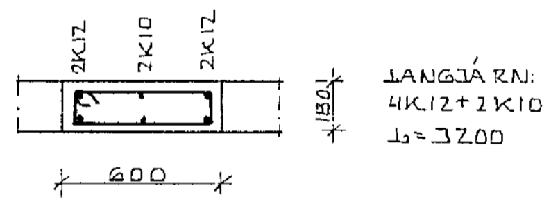
SNIB A-A 1:20 SNIB B-B 1:20 SNIB C-C 1:20 SNIB D-D 1:20
