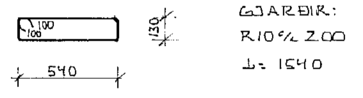
SNIB Í SÚLU S1 1:20
