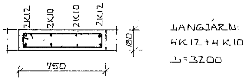
SNIB Í SÚLU S1 1:20
