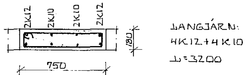
SNIB Í SÚLU S1 1:20
