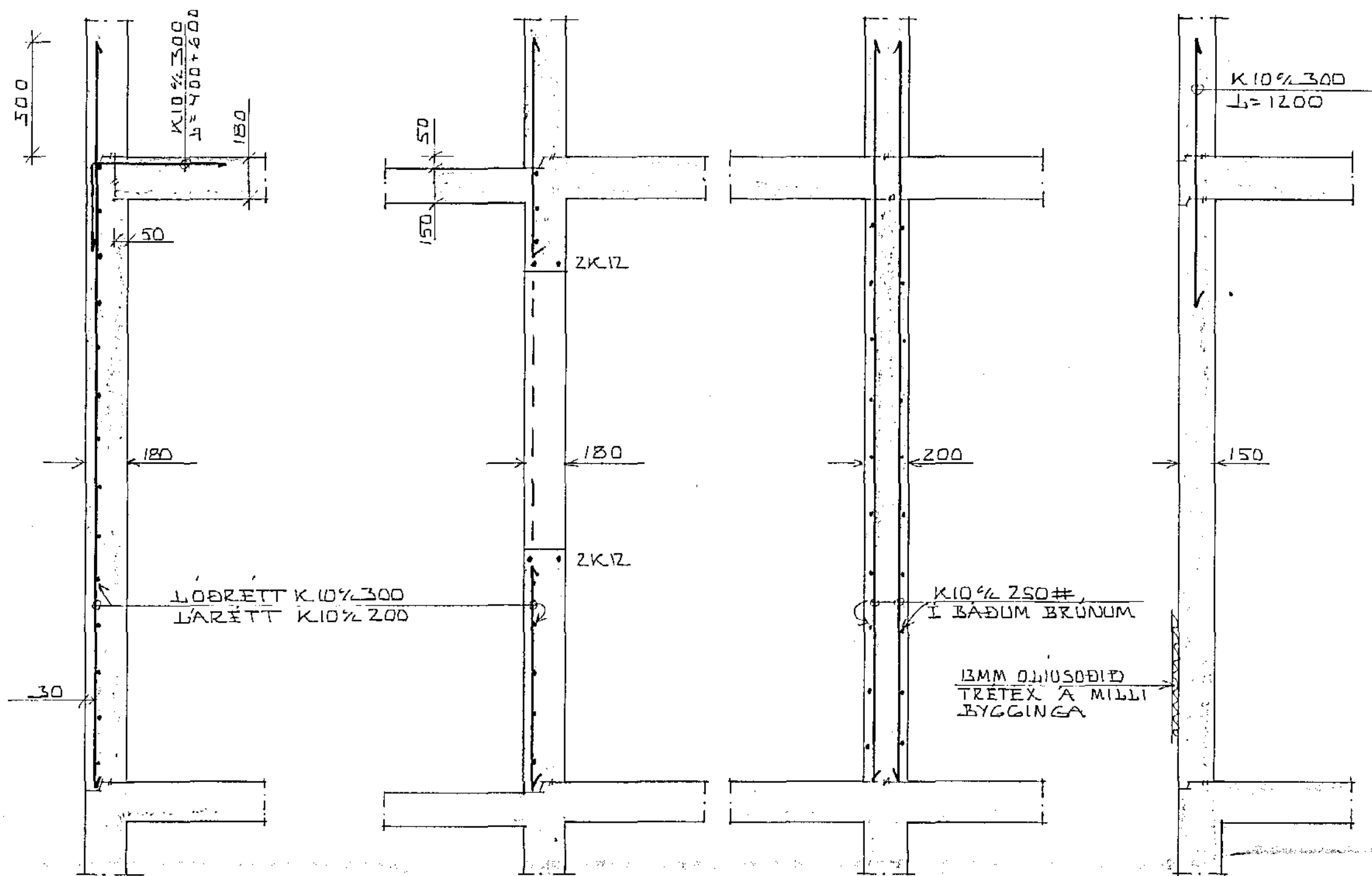
SNIB A-A 1:20 SNIB B-B 1:20 SNIB C-C 1:20 SNIB D-D 1:20
