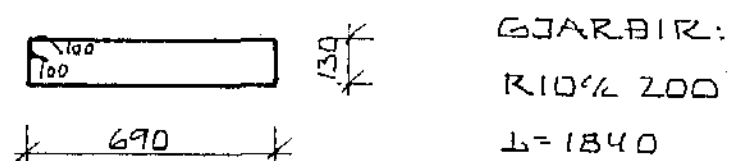
SNIB Í SÚLU S3 1:20
