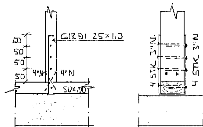
SÉRMYND - III 1:10
