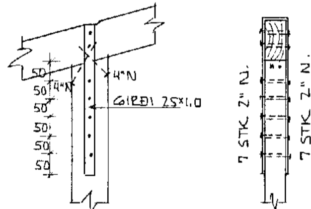
SÉRMYND - IV 1:10
