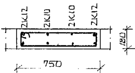
SNIB Í SÚLU S1 1:20
