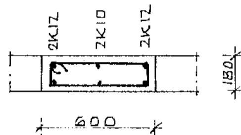
SNIB A-A 1:20 SNIB B-B 1:20 SNIB C-C 1:20 SNIB D-D 1:20
