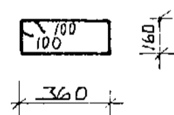
SNIB Í SÚLU S2 1:20
