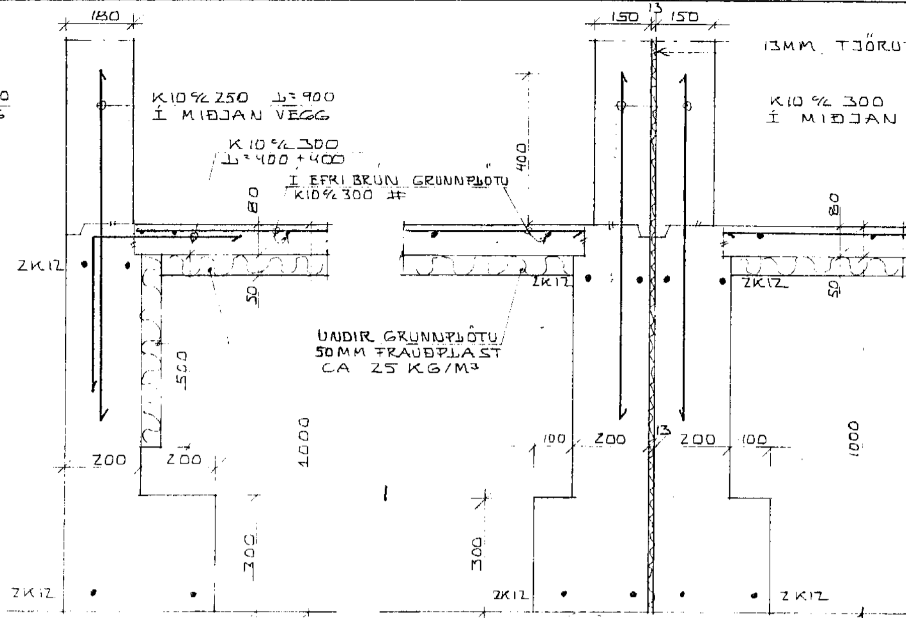
SNID B-B 1:10
