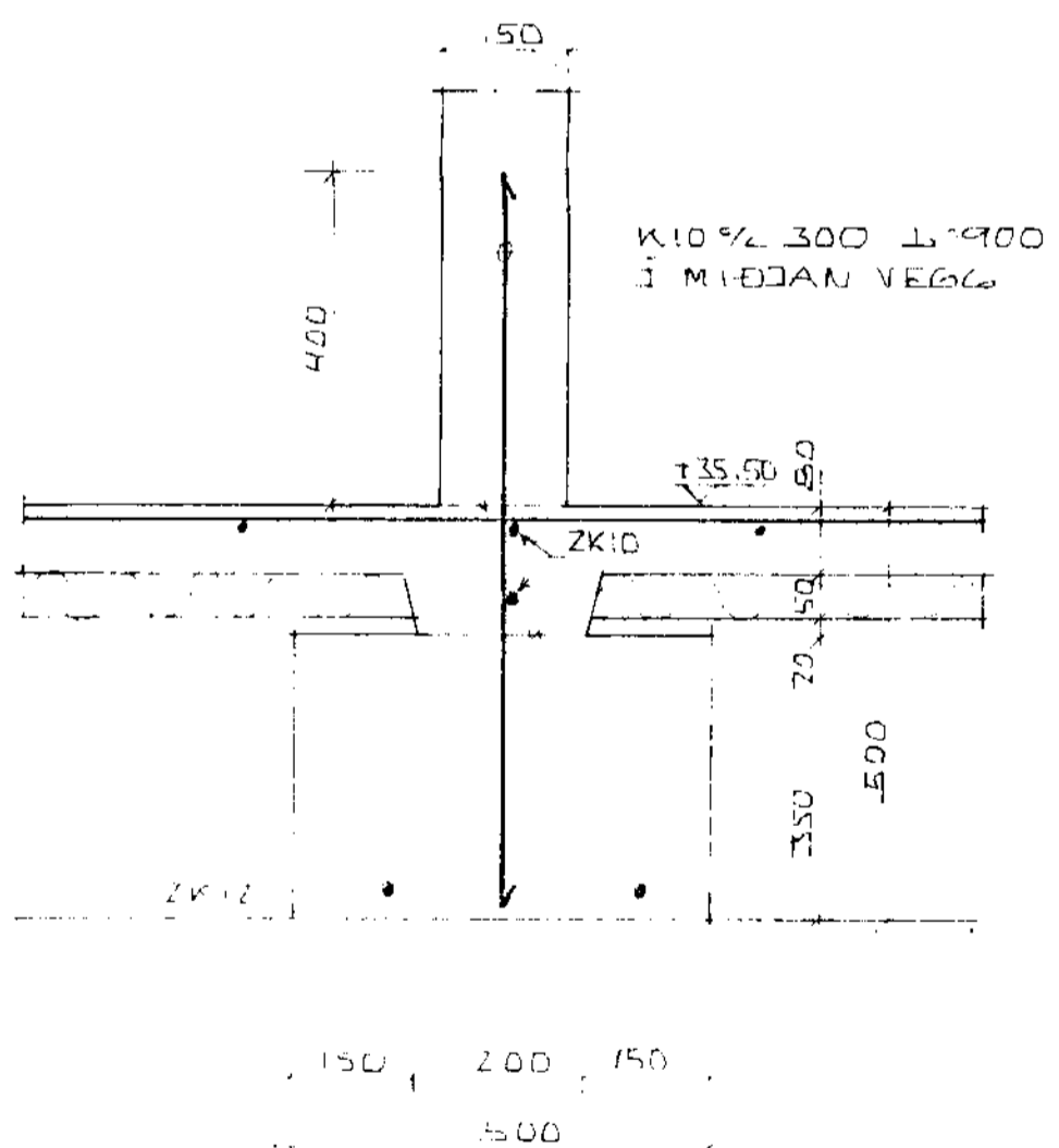
SNID A-A 1:10
