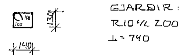
SNID I SÚLU S6 1:20
