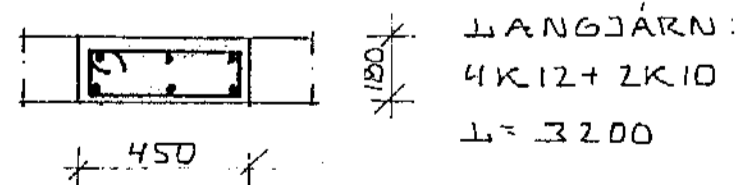
SNID I SÚLU S2 1:20
