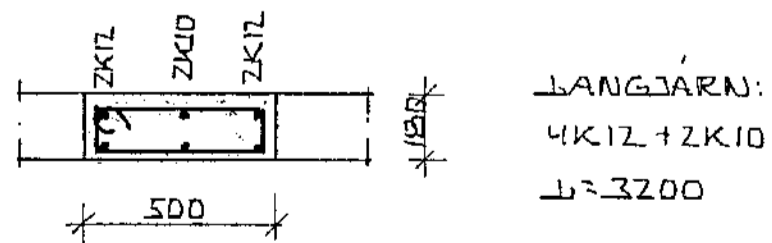
SNID I SÚLU S1 1:20
