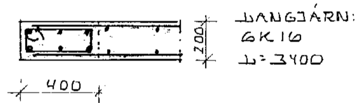
SNID A-A 1:20 SNID B-B 1:20 SNID C-C 1:20 SNID D-D 1:20 SNID E-E 1:20
