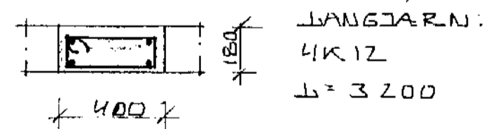
SNID I SÚLU S6 1:20
