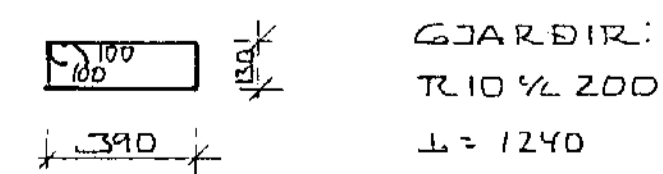
SNID I SÚLU S4 1:20
