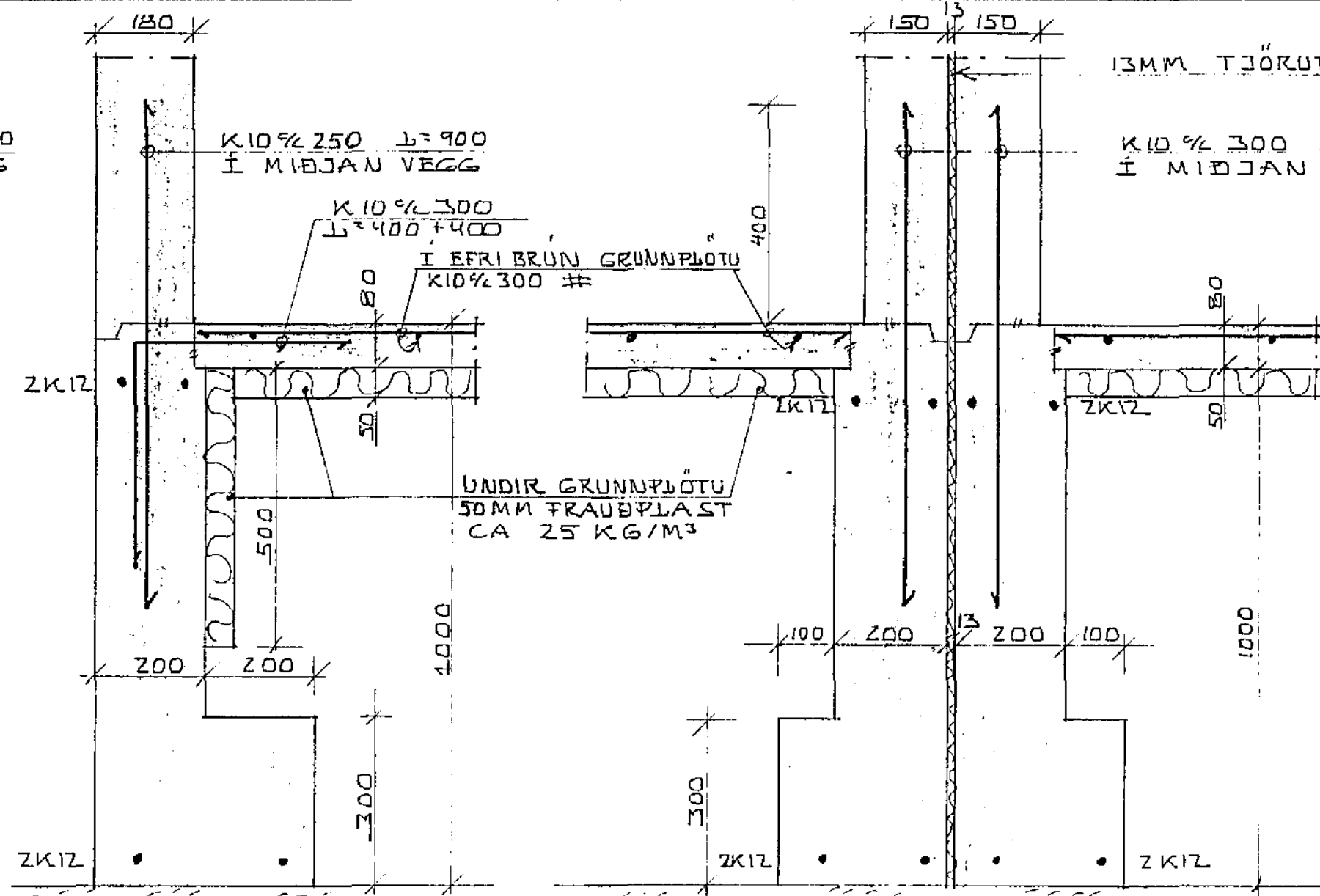
SNID B-B 1:10
