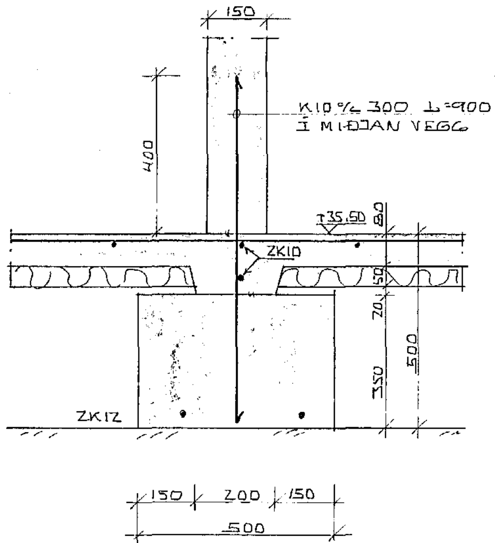
SNID A-A 1:10
