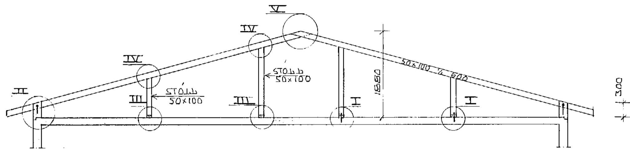
SNIB A-A 1:50
