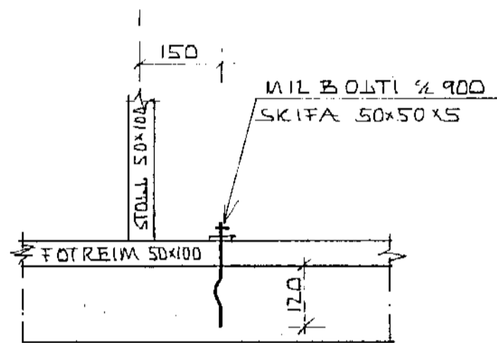
FESTING FÓTREIMA
