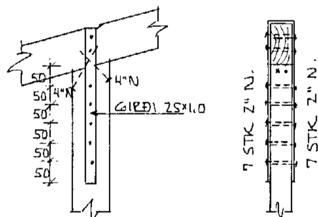
SÉRMYND - IV 1:10
