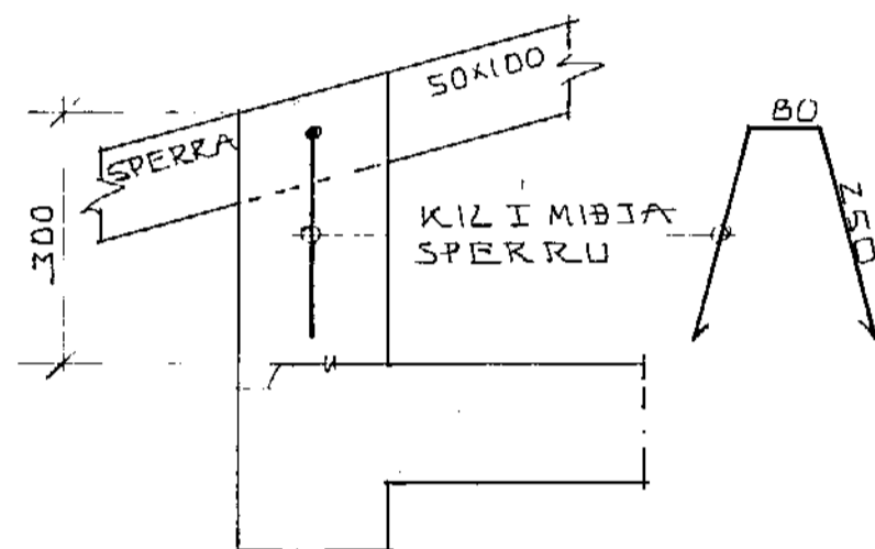
SÉRMYND - II 1:10
