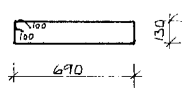
SNIB Í SÚLU S3 1:20
