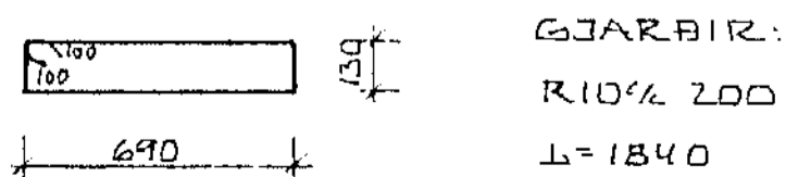
SNIB Í SÚLU S3 1:20
