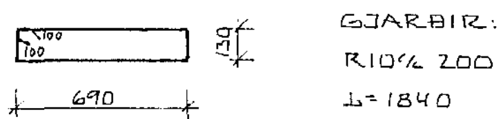
SNIB Í SÚLU S3 1:20
