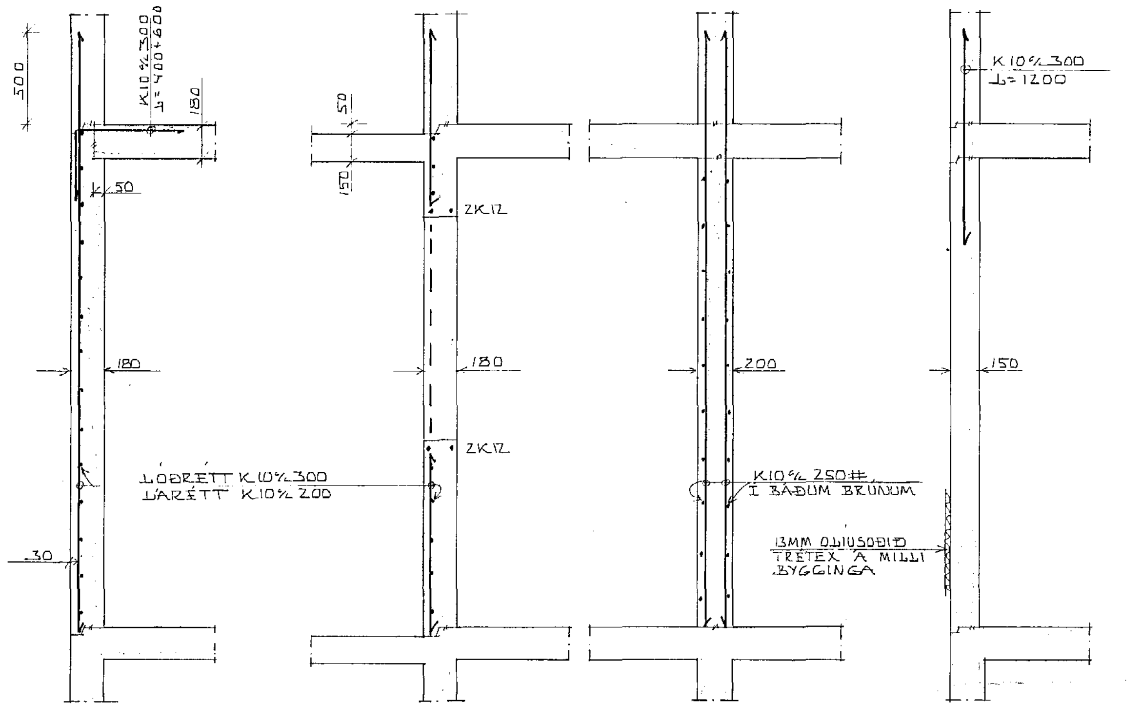
SNIB A-A 1:20 SNIB B-B 1:20 SNIB C-C 1:20 SNIB D-D 1:20
