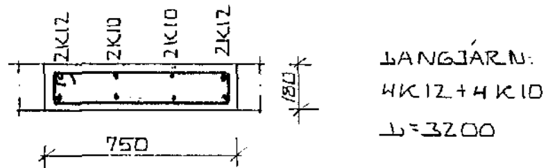
SNIB Í SÚLU S1 1:20
